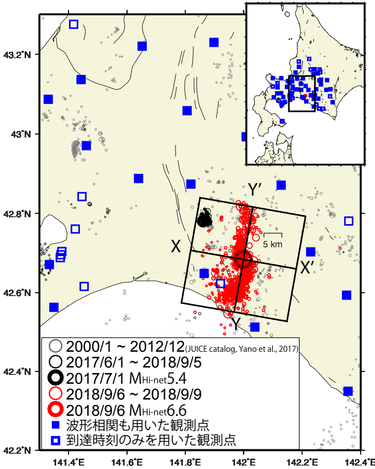
図1 平成30年北海道胆振東部地震の震源周辺における震央分布。短形領域内(右上)の深さ50km以浅の地震について防災科研Hi-net(自動処理を含む)の震源を波形相関データを用いたDouble-Difference法(DD法, Waldhasuer and Ellsworth, 2000)により再決定した。
