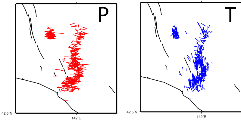
図4 防災科研Hi-net初動解によるP(左)とT(右)軸の分布。手動検測によるM>1.5のPとT軸を、それぞれ再決定した震源位置に示す。
