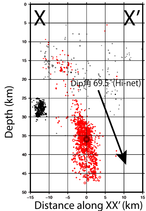
図3 X-X'に沿った矩形領域内の震源の深さ分布。防災科研Hi-net初動解のうち横ずれ断層型のDip角も示す。
