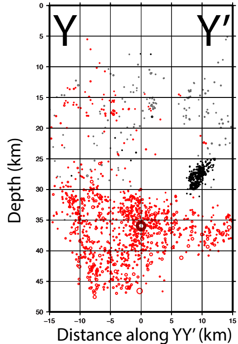
図2 Y-Y'に沿った矩形領域(図1の主地図上)内の震源の深さ分布。走向は10°。
