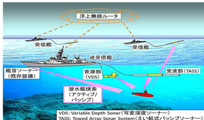
可変深度ソーナーシステムの運用のイメージ
