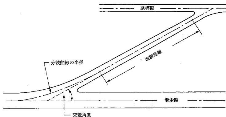
図-3.7.1 高速離脱誘導路の標準平面形状
