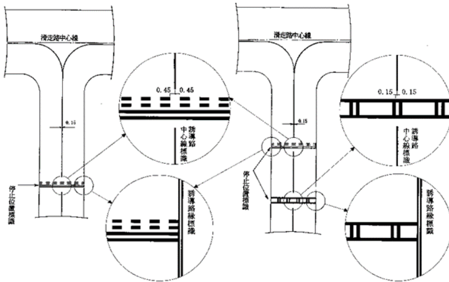
図-3.12.8 停止位置標識と誘導路中心線及び誘導路縁標識の関係
