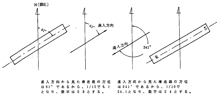
図-3.12.1 指示標識の例
