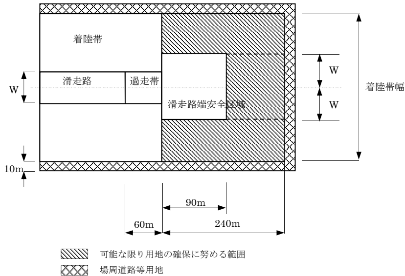
図-3.6.1 コード番号が4の精密進入用滑走路の場合
