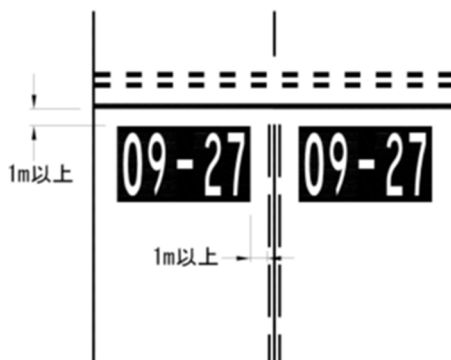
図-3.12.10 停止位置案内標識と誘導路中心線標識及び停止位置標識との関係
