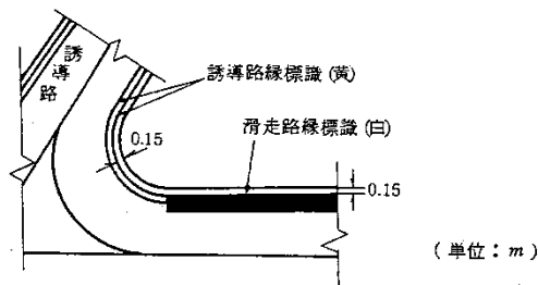
図-3.12.4 誘導路縁標識と滑走路縁標識の接続の例
