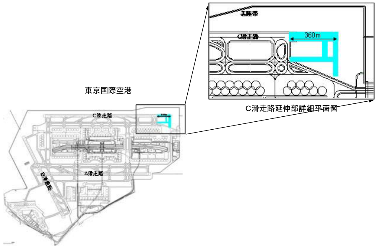
図一2 C滑走路延伸区域
