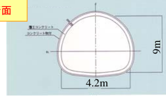
分水路取水庭
