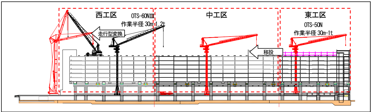
図-5 タワークレーン設置計画図
