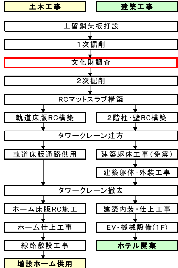
図-3 施工フロー図
