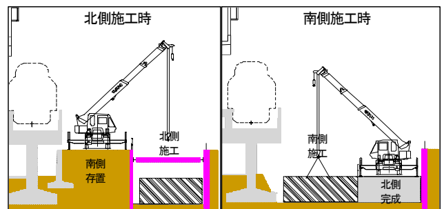
図-4 マットスラブ分割施工要領図
