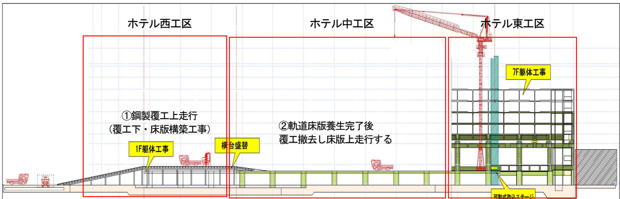
図-6 鋼製覆工設置計画図
