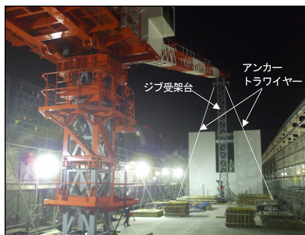
写真-2 タワークレーン台風対策状況
