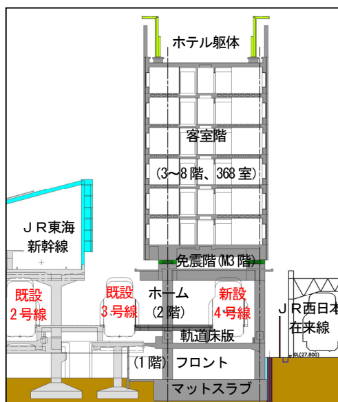
図-2 ホーム・ホテル断面図
