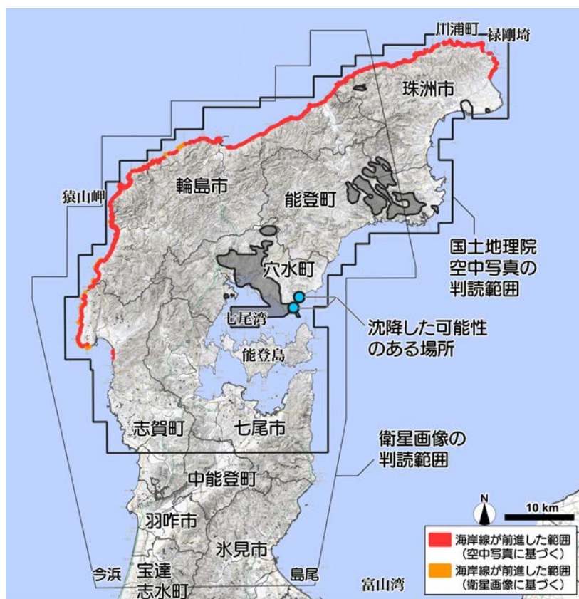
図1 判読範囲と地震後に陸化した範囲
