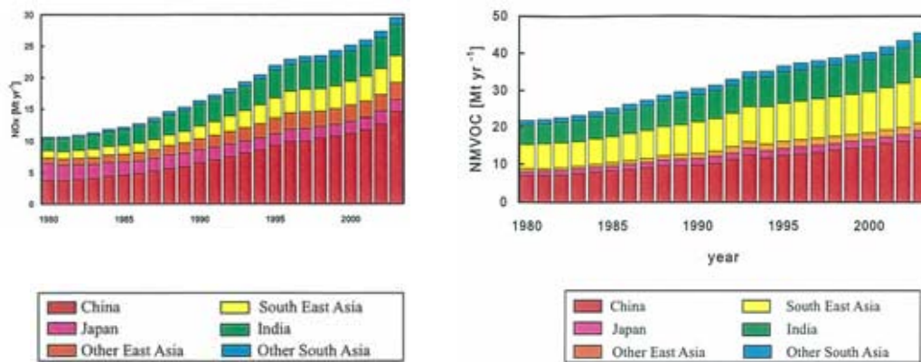
図 2-2 アジア全体の NO x 及び NMVOC 排出量推計値(Ohara et al.,2007a)
