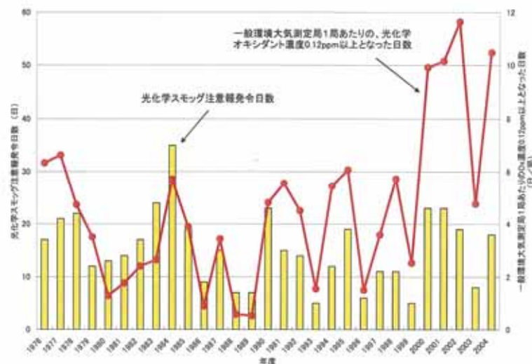
図1-8 東京都における光化学スモッグ注意報発令日数と、一般環境大気測定局1局あたりのオキシダント濃度0.12ppm以上となった日数の経年変化(ただし、2004年度は12月末までの値)(東京都,2005,東京都環境局環境改善部,2005)
