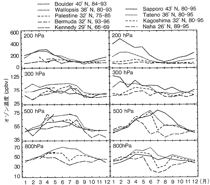
図 1-23 米国、西部大西洋、日本における高度別オゾンの季節変化 ( Boulder : 米国コロラド州 ( 米国西側 ) Wallopsis ( Wallops Island ): 米国バージニア州 ( 米国東側 ) Palestine : 米国テキサス州 ( 米国中央 ) Bermuda : バミューダ ( 西部大西洋 ) Kennedy : 29 ° N、31 ° W、Sapporo : 札幌、Tateno : 館野、Kagoshima : 鹿児島、Naha : 那覇(Logan,1999 , 秋元ほか編,2002)
