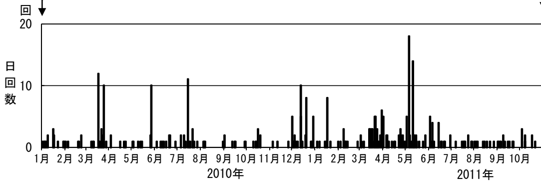
図7※ 岩手山 日別地震回数（2010年1月～2011年10月）
