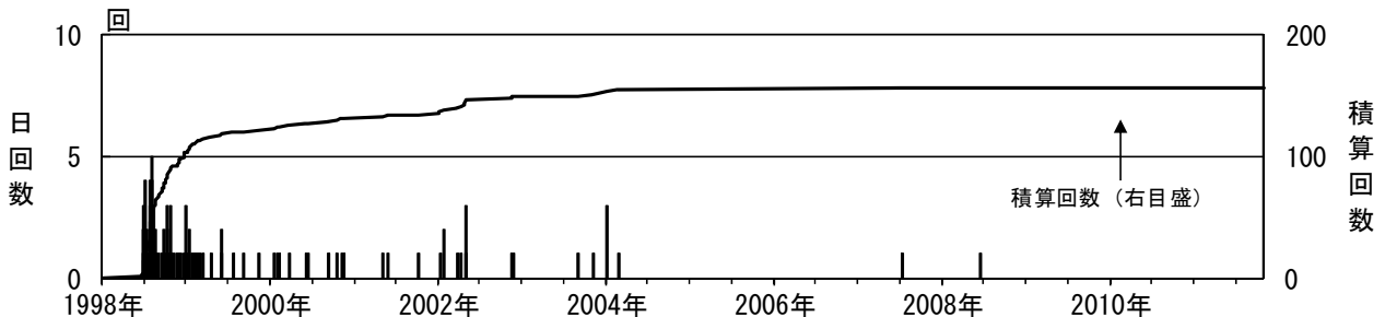
図8※ 岩手山 日別微動回数（1998年1月～2011年10月）
