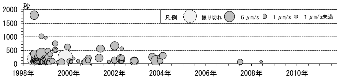
図9※ 岩手山 微動の継続時間と上下動最大振幅（1998年1月～2011年10月）
