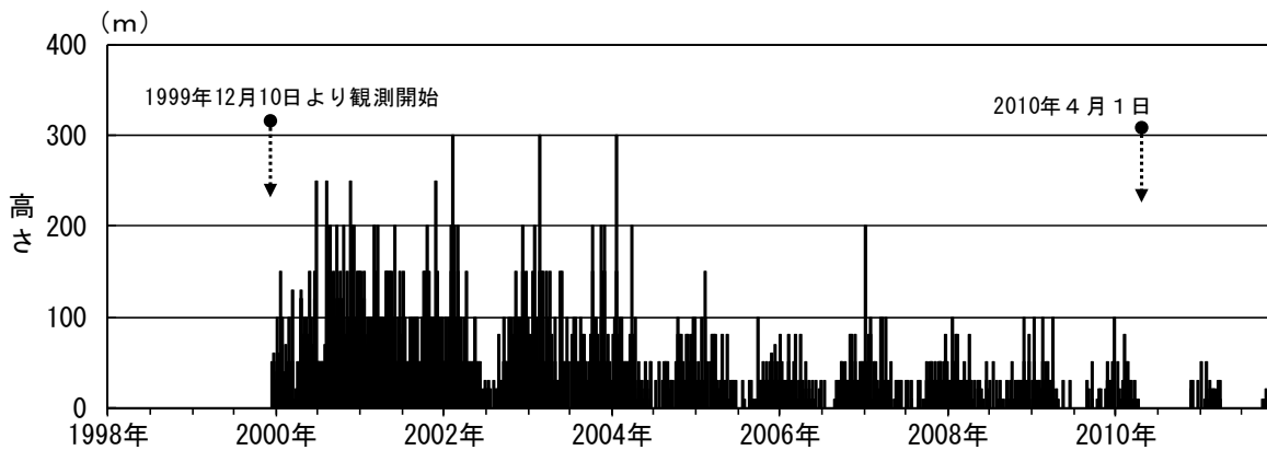
図3 岩手山 日最大噴気の高さ（1999年12月～2011年10月） 柏台遠望カメラで、1999年12月10日より観測を開始しています。 2010年3月までは、黒倉山のみを観測していましたが、2010年4月1日より、岩手山全体を観測しています。
