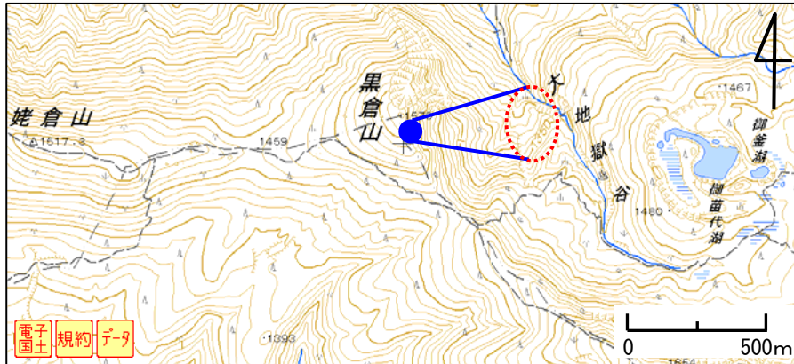
図4 岩手山 図5の可視画像及び地表面温度分布 1) 撮影位置
