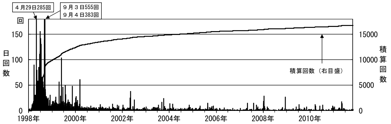
図6※ 岩手山 日別地震回数（1998年1月～2011年10月）
