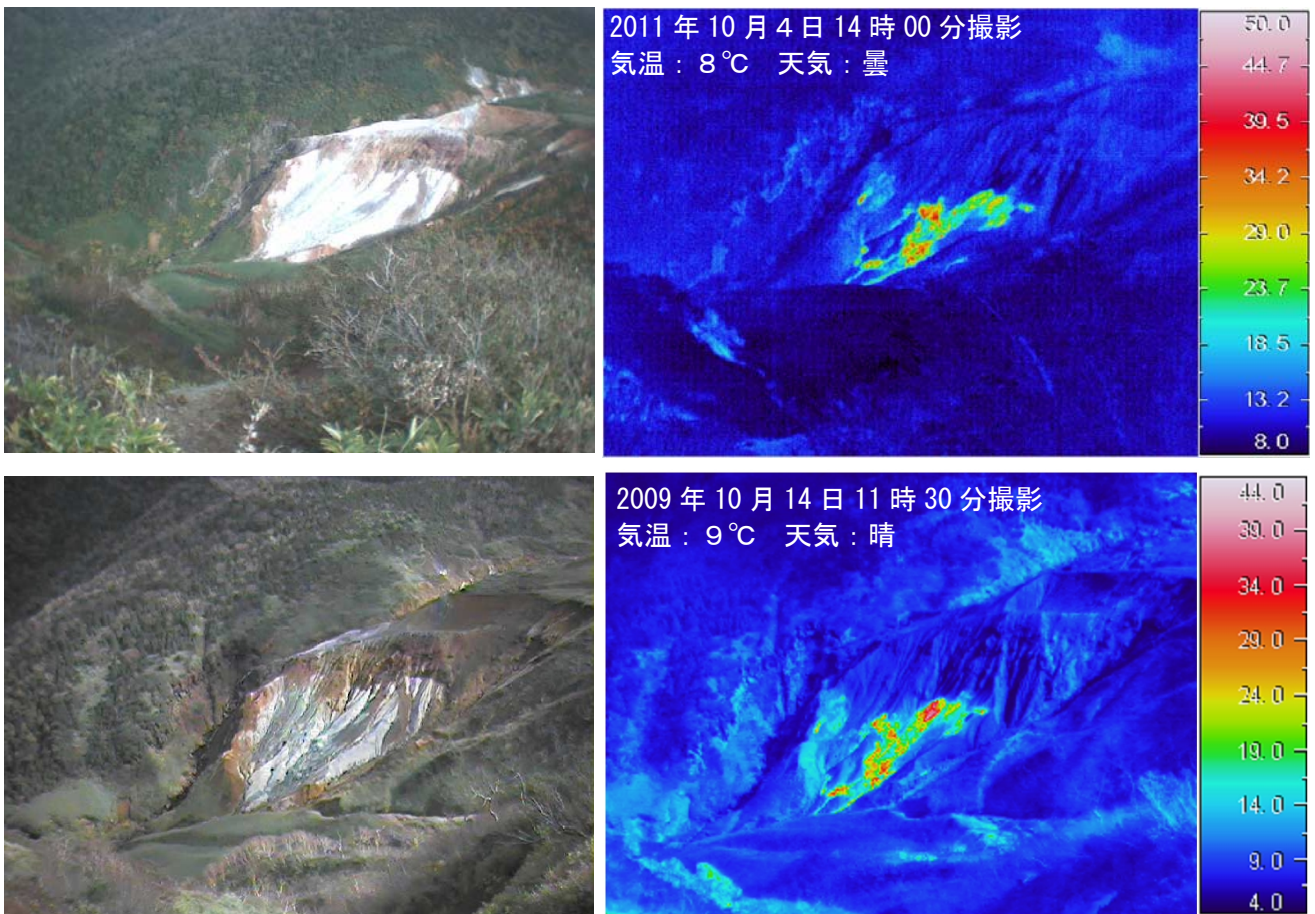
図5 岩手山 大地獄谷の可視画像 (左) と地表面温度分布 1) (右) 上段：2011年10月4日、下段：2009年10月14日
