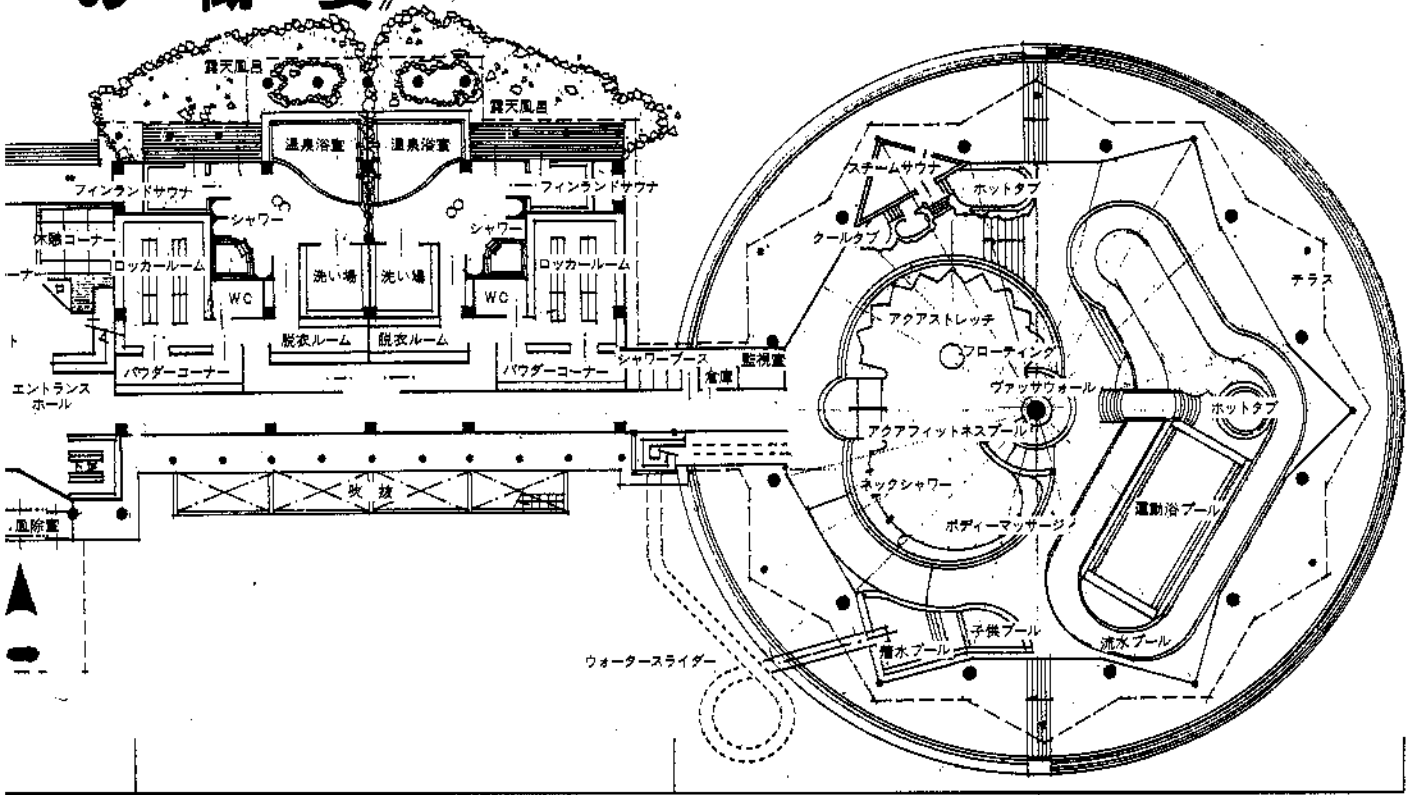
一階平面図
