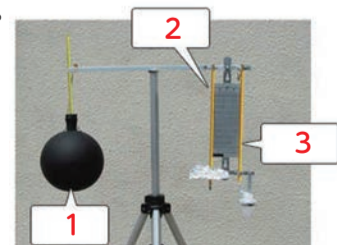
▲WBGT値測定器。1、2、3それぞれの温度を測り、「気温」とは異なる「暑さ」の指数を測る。(環境省熱中症予防情報サイトの写真を加工)
