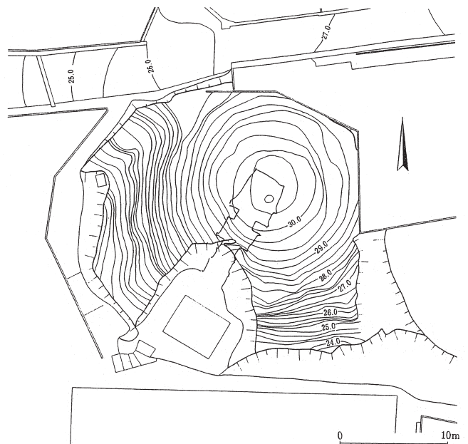
福岡市博多区金隈 今里不動古墳墳丘測量図
