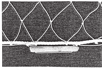
棒状土錘装着法復元
