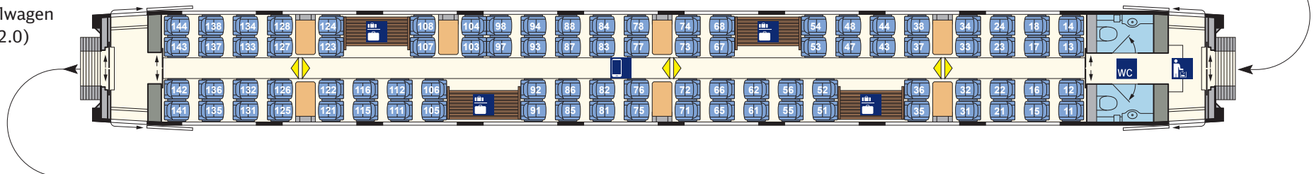
2. Kl.-Mittelwagen (Bpmz 2412.3) Nr. 6
