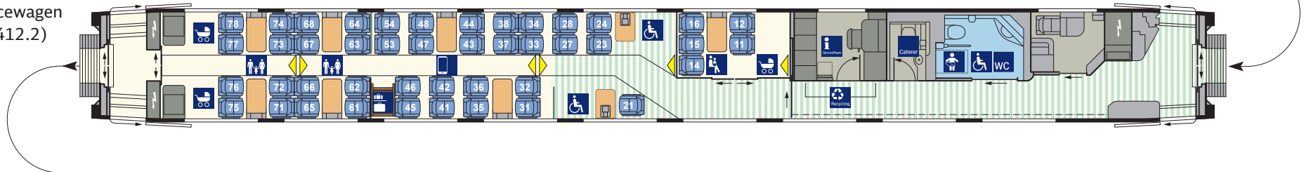
2. Kl.-Mittelwagen (Bpmz 3412.2) Nr. 24/34
