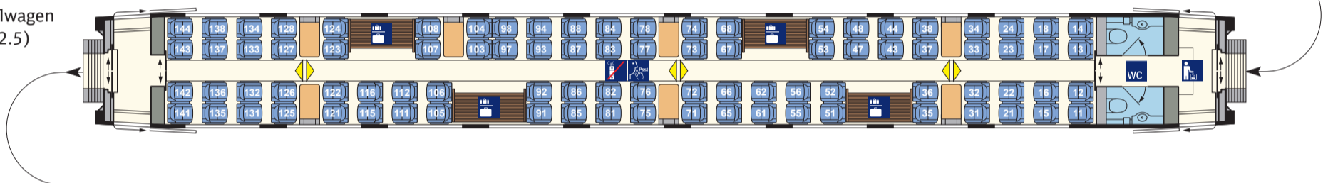
2. Kl.-Mittelwagen (Bpmz 2412.8) Nr. 2
