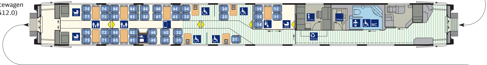
2. Kl.-Mittelwagen (Bpmz 9812.0) Nr. 7
