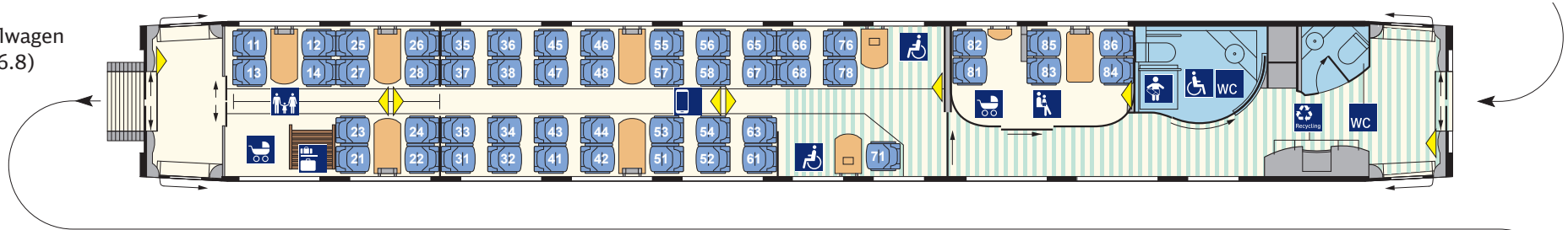
2. Kl.-Mittelwagen (Bpmz 406.7) Nr. 23/33
