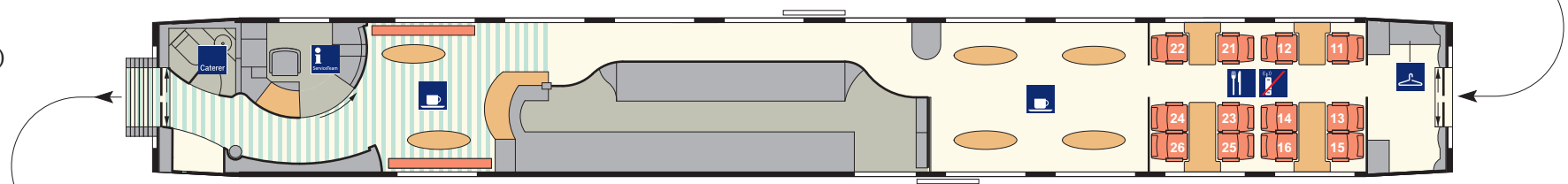
Bordbistro (BRmz 406.3) Nr. 26/36
