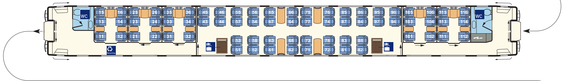
2. Kl.-Wagen (Bvmmz 188)
