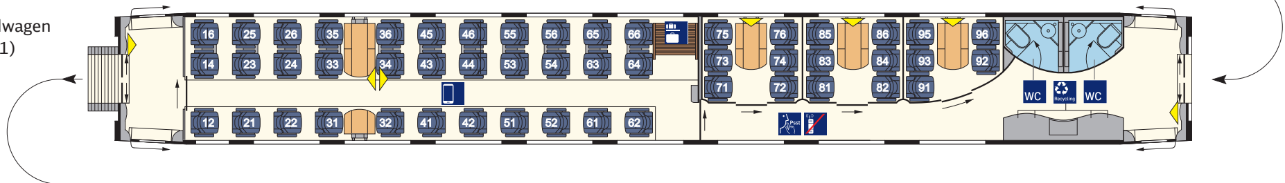
2. Kl.-Mittelwagen (Bpmz 403.2) Nr. 27/37
