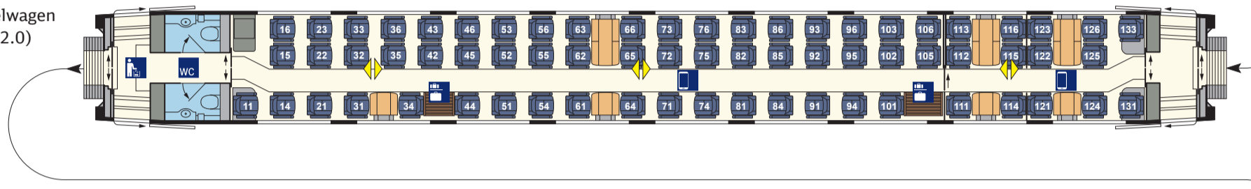
1. Kl.-Mittelwagen (Apmzf 1412.0) Nr. 11
