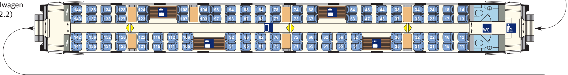
2. Kl.-Mittelwagen (Bpmz 3412.7) Nr. 22/32
