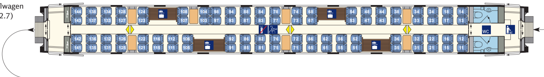
2. Kl.-Endwagen (Bpmdzf 7812.2) Nr. 21/31
