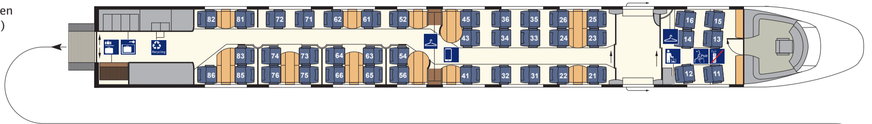
Bordbistro/2. Klasse (BRpmz 415.1) Nr. 27/37
