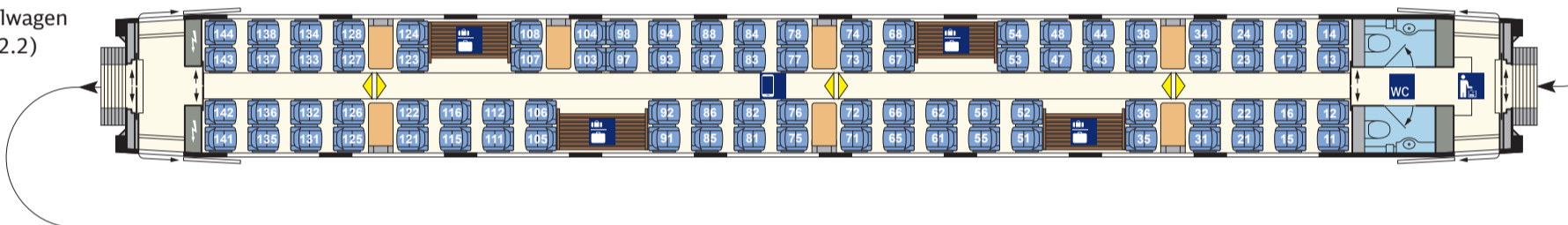
2. Kl.-Mittelwagen (Bpmz 3812.2) Nr. 23/33
