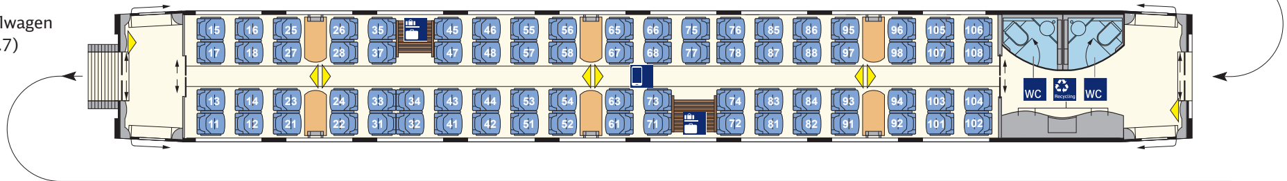
2. Kl.-Mittelwagen (Bpmz 403.6) Nr. 22/32
