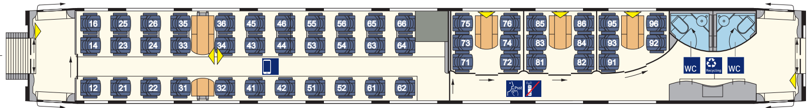
1. Kl.-Mittelwagen (Avmz 406.1) Nr. 28/38
