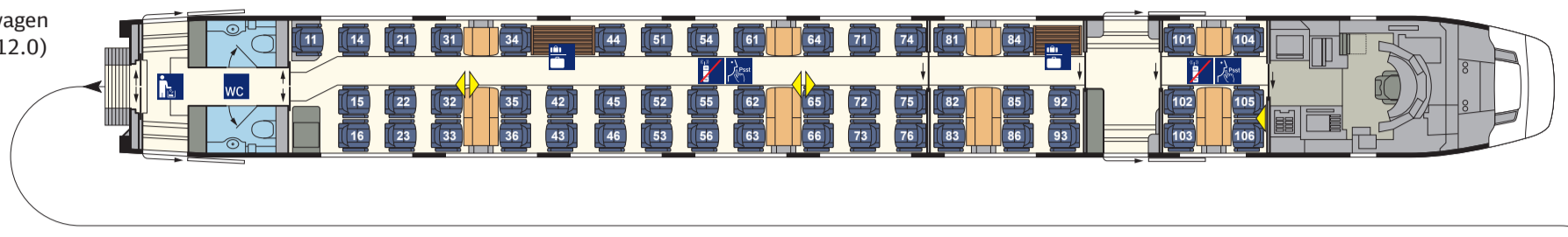
1. Kl.-Mittelwagen (Apmzf 1812.0) Nr. 12
