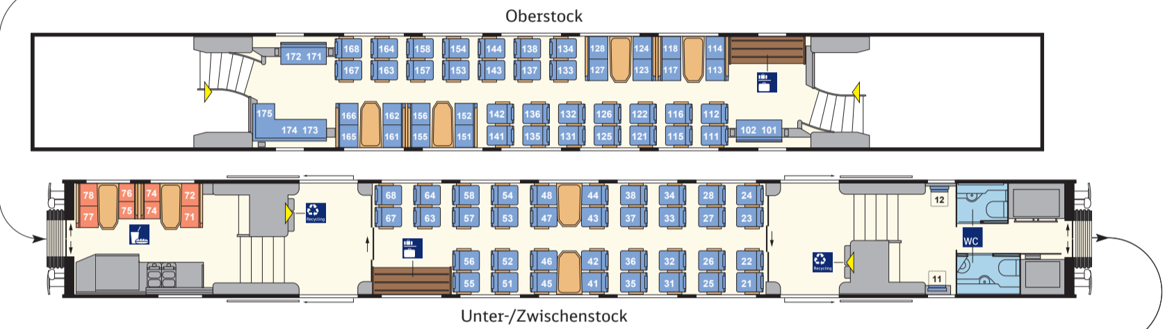
2. Kl.-Mittelwagen (DBpza 110.E) Nr. 5
