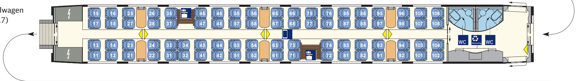
2. Kl.-Mittelwagen (Bpmz 406.6) Nr. 22/32
