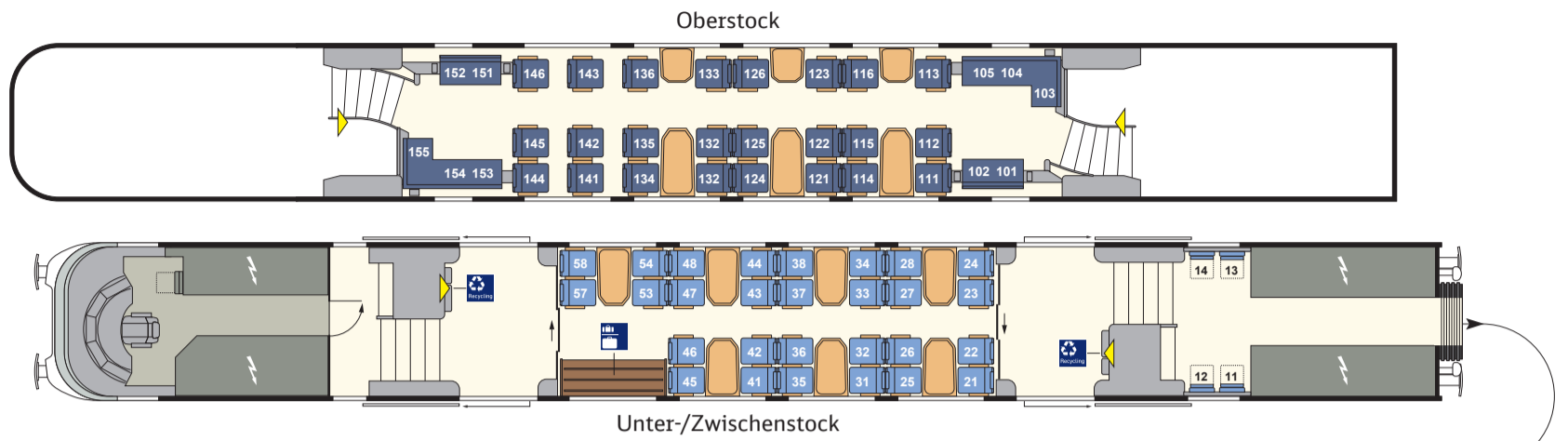
1./2. Kl.-Endwagen (DABpzfa 110.F) Nr. 6
