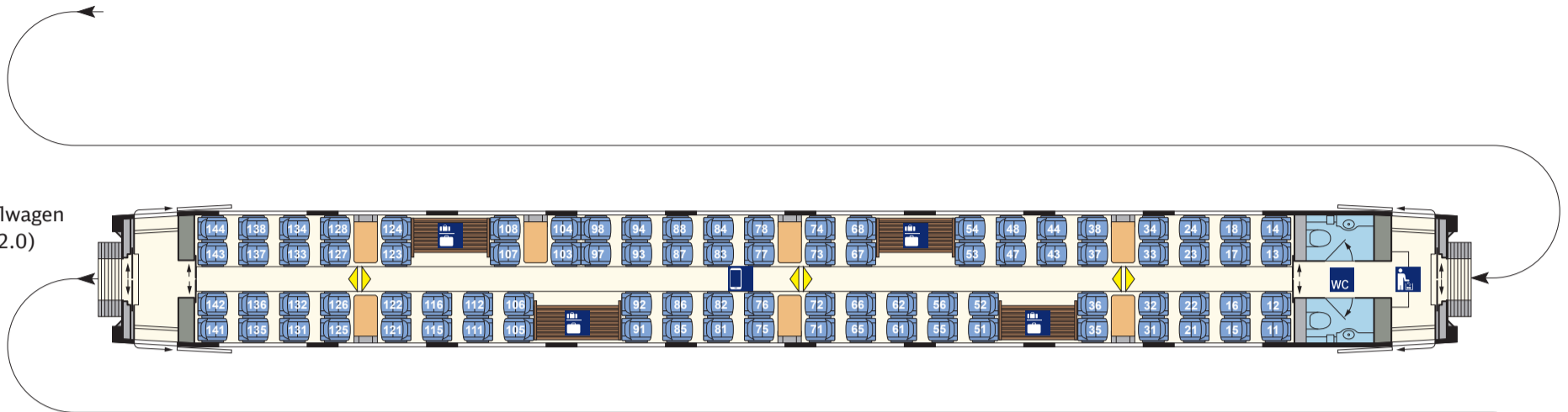
2. Kl.-Mittelwagen (Bpmz 2412.5) Nr. 3
