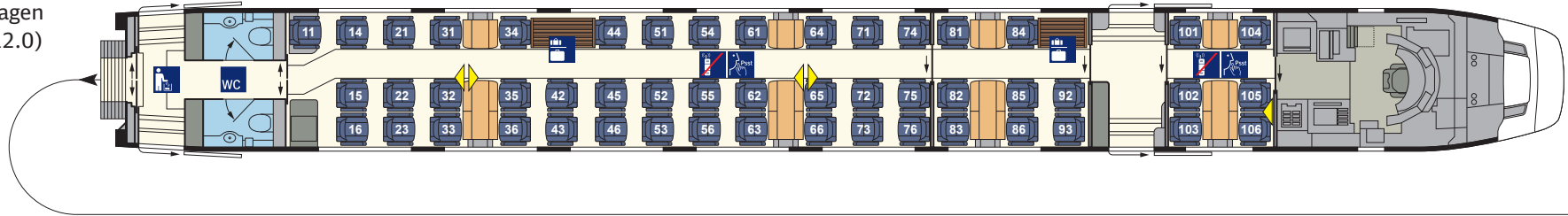
1. Kl.-Mittelwagen (Apmz 1812.0) Nr. 12
