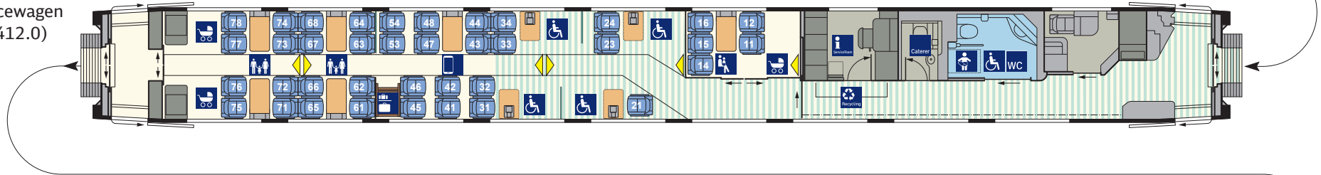
2. Kl.-Mittelwagen (Bpmz 9812.0) Nr. 8
