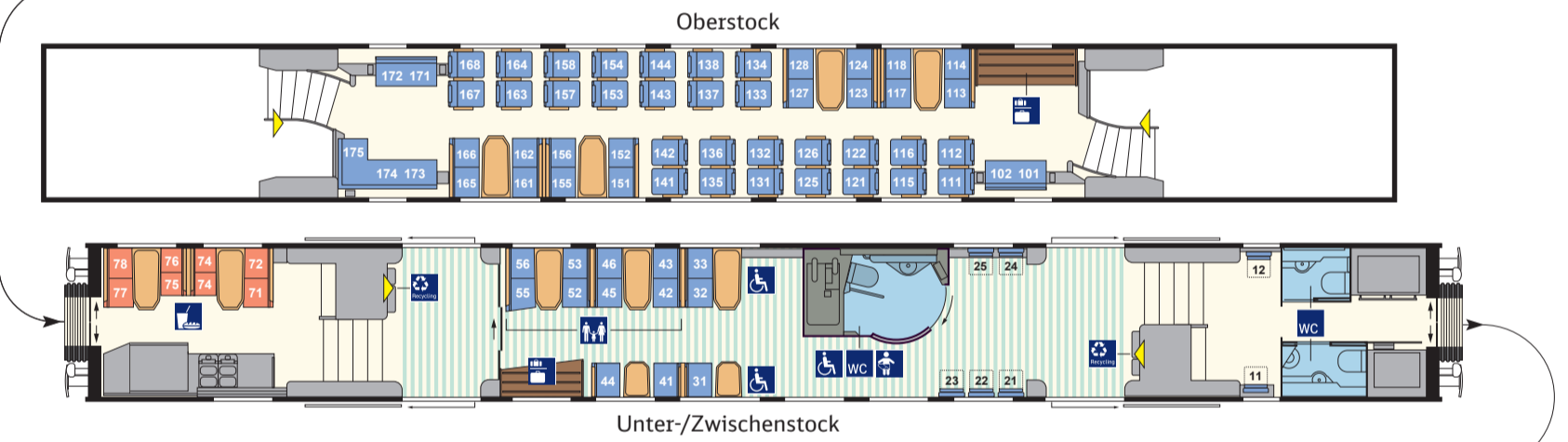
2. Kl.-Mittelwagen (DBpbza 110.D) Nr. 4
