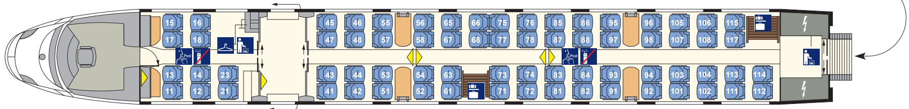
2. Kl.-Endwagen (Bpmzf 403.5) Nr. 21/31
