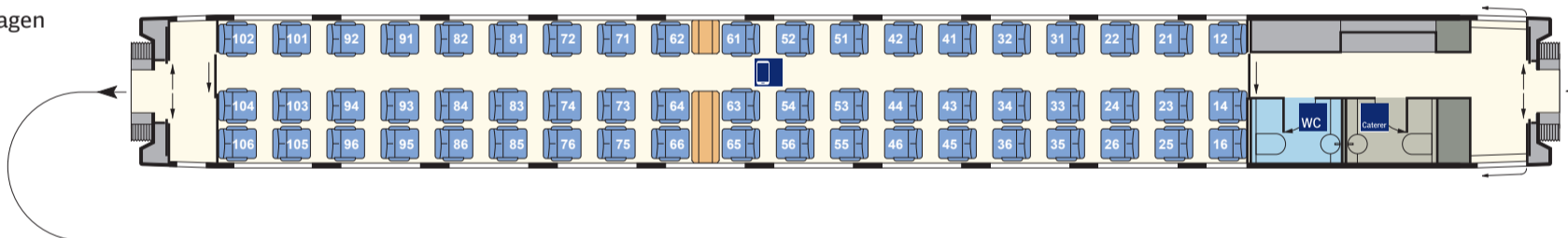
Bordbistro/1. Klasse (Apmkz 116.6) Nr. 6
