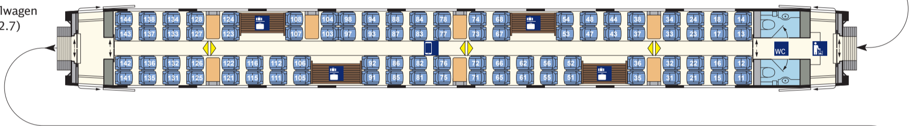
2. Kl.-Mittelwagen (Bpmz 2412.5) Nr. 3
