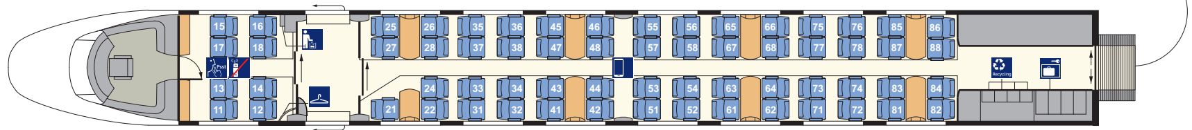
2. Kl.-Endwagen (Bpmzf 411.5) Nr. 21/31
