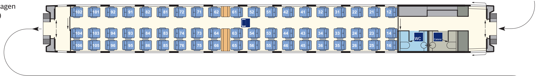
Bordbistro/1. Klasse (Apmkz 116.6) Nr. 6
