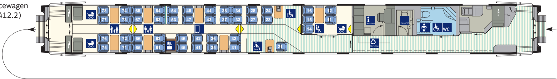
2. Kl.-Mittelwagen (Bpmz 3412.2) Nr. 24/34
