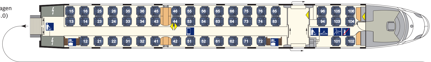
1. Kl.-Mittelwagen (Avmz 403.1) Nr. 28/38
