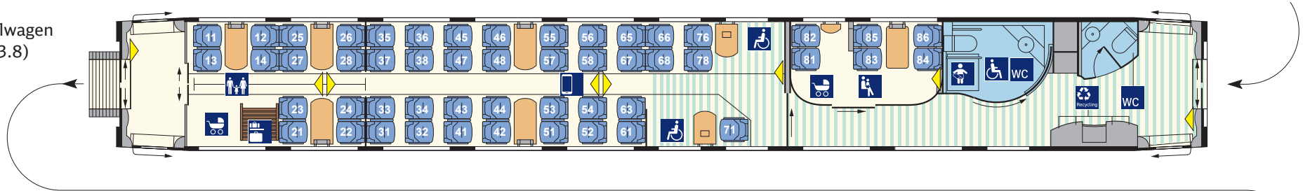
2. Kl.-Mittelwagen (Bpmz 403.7) Nr. 23/33
