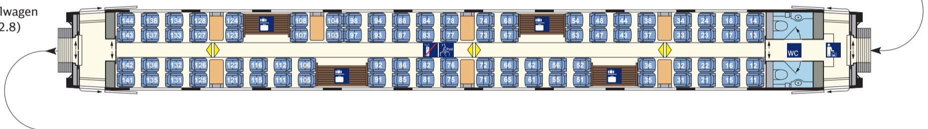
2. Kl.-Endwagen (Bpmdzf 5812.0) Nr. 1
