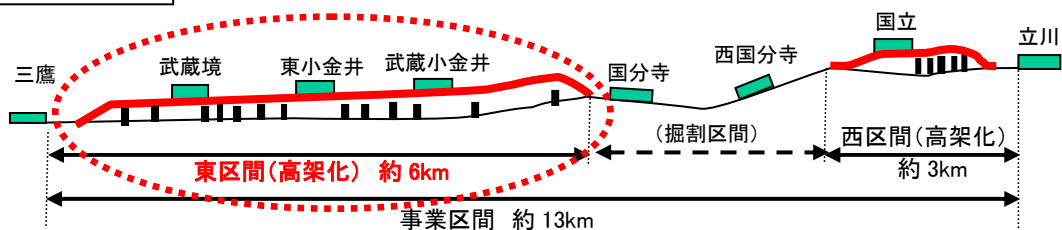
高架化後断面図
