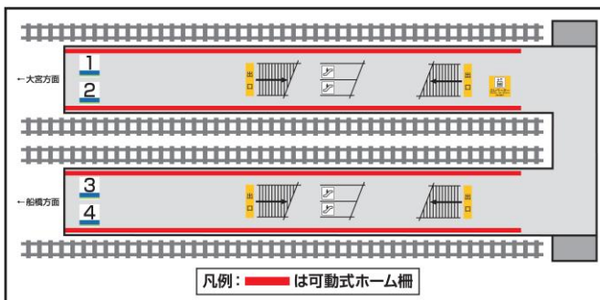
△柏駅 可動式ホーム柵設置図
