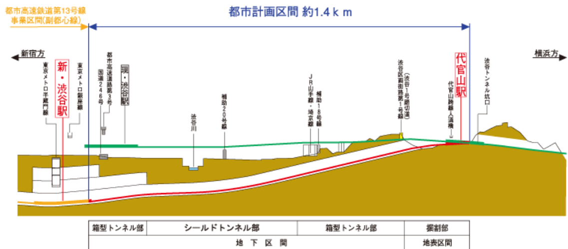
縦断面図
