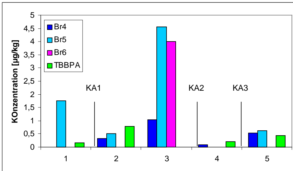
Abb. 13: PBDE und TBBPA in Oberflächensedimenten der Körch (Angaben in µg/kg Trockengewicht; KA1: Möhringen, KA2: Plieningen, KA3: Denkendorf)
