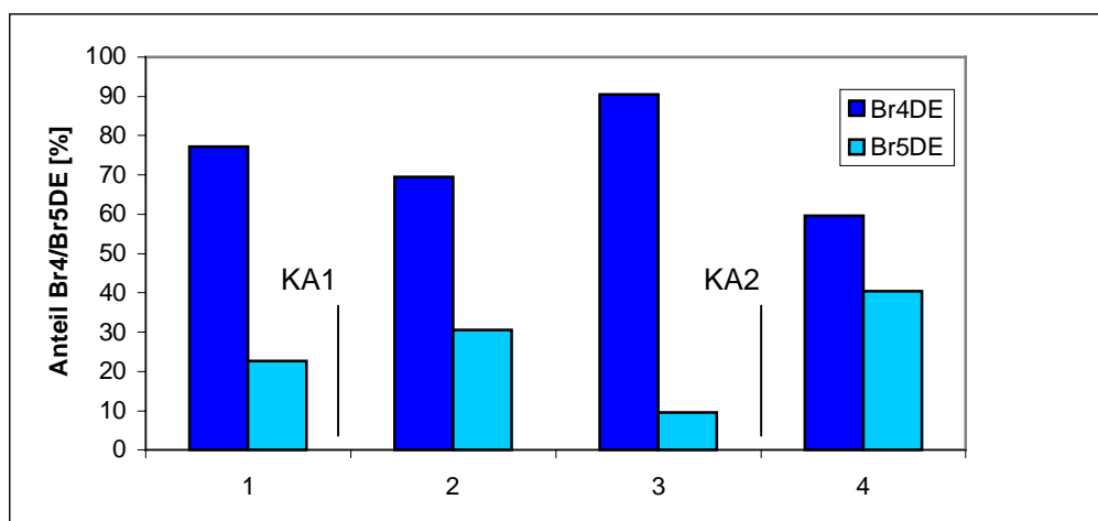
Abb. 14: Verhältnis der Br4DE und Br5DE in Sedimenten des Neckars; Angaben in Prozent des Gesamtgehalts (KA1: Bad Niedernau, KA2: Tübingen)
