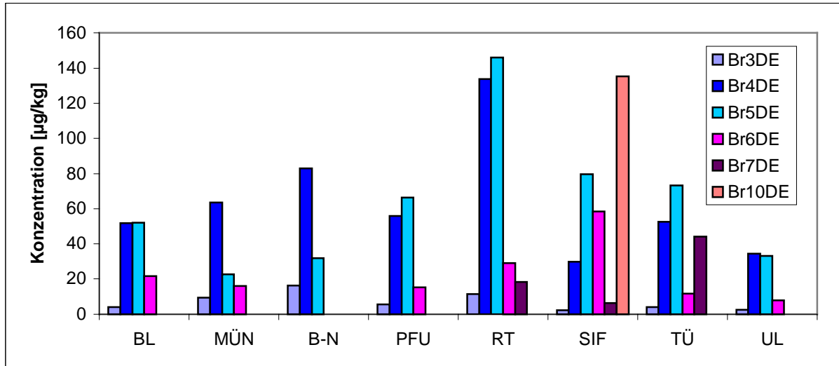
Abb. 16: PBDE-Konzentrationen und –verteilungen in Klärschlämmen (Angabe in µg/kg)
