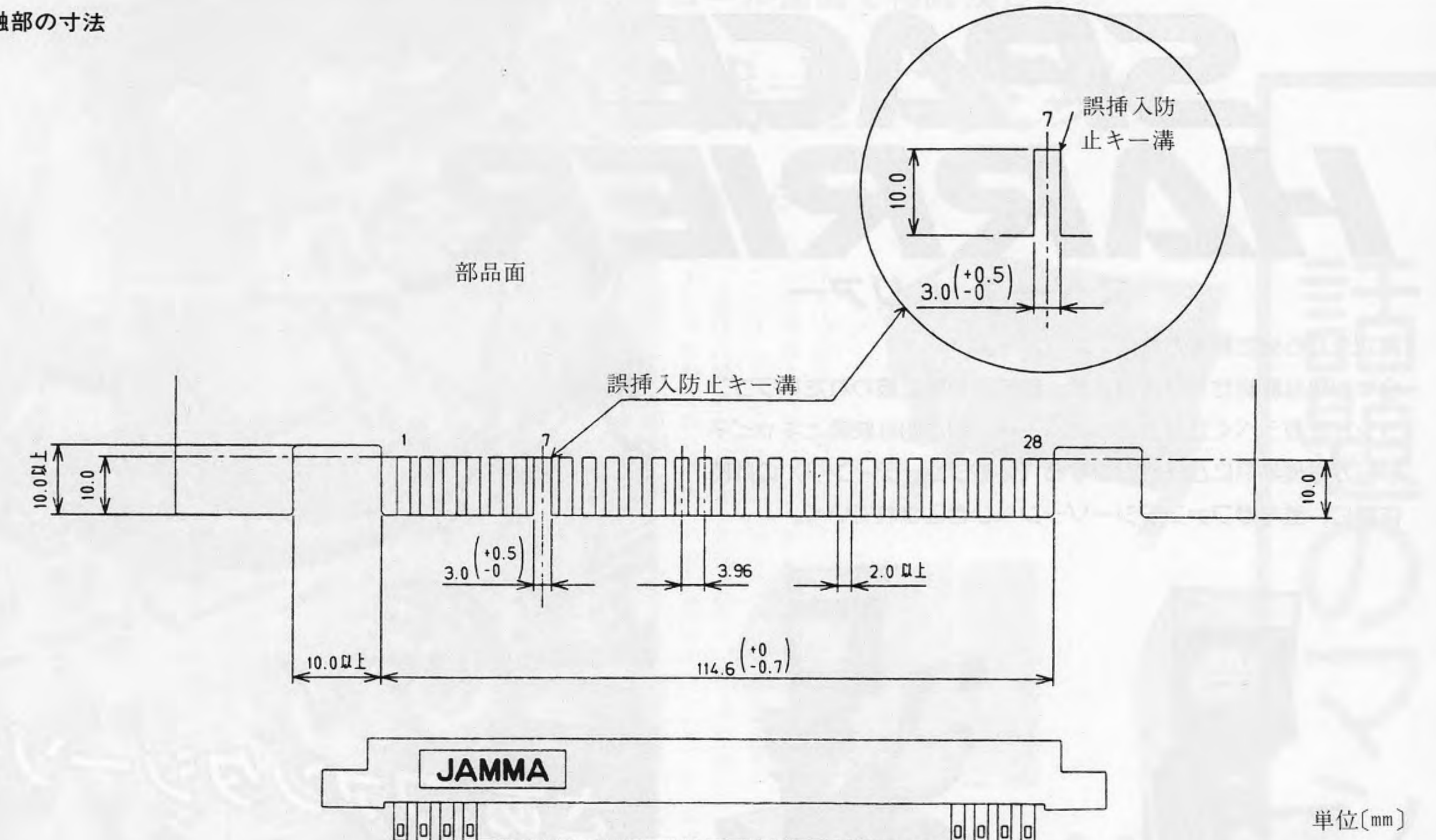
図2 メイン基板の寸法測定箇所
