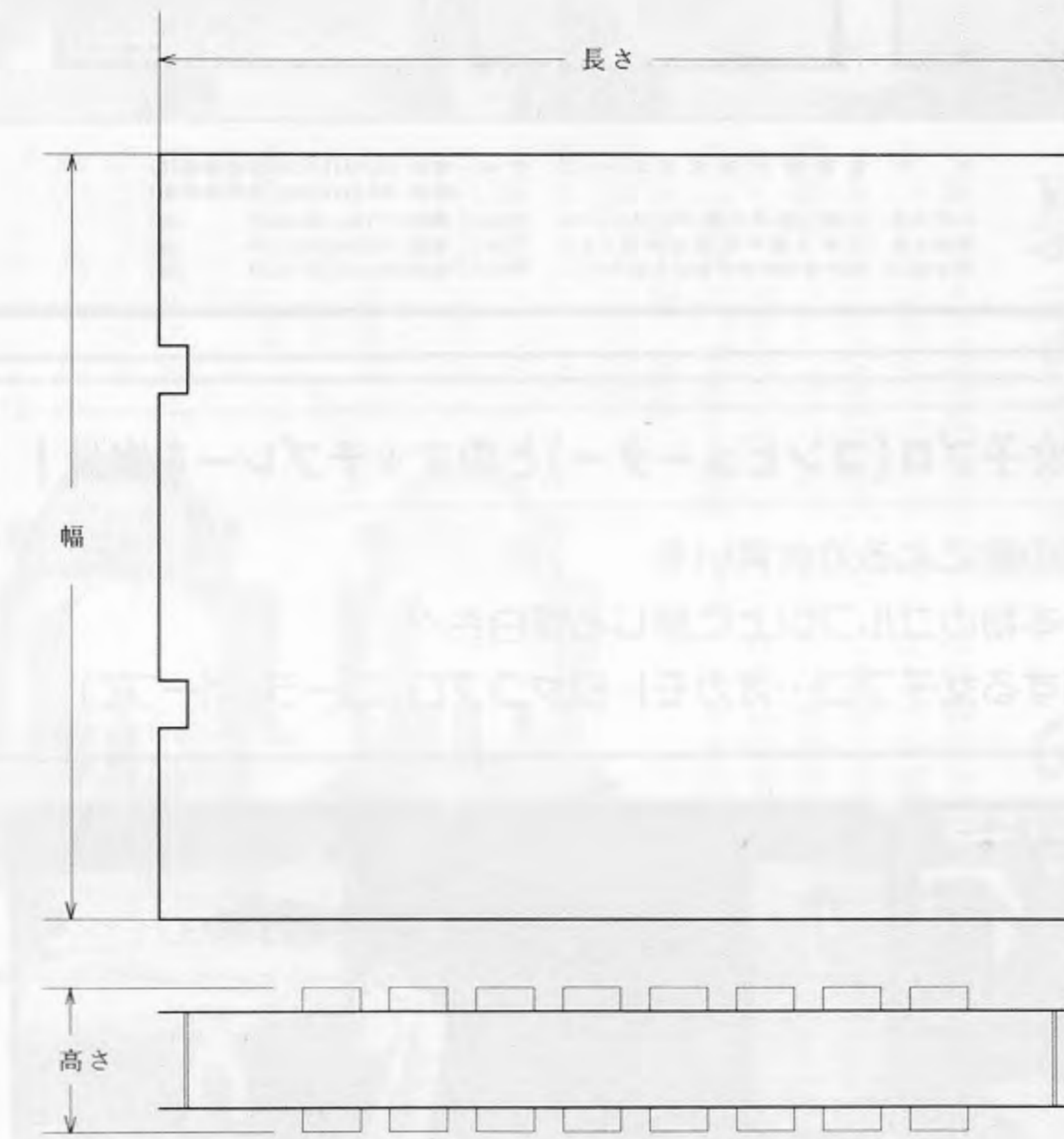
図2 メイン基板の寸法測定箇所
