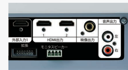
HDMI出力2系統、入力1系統装備
