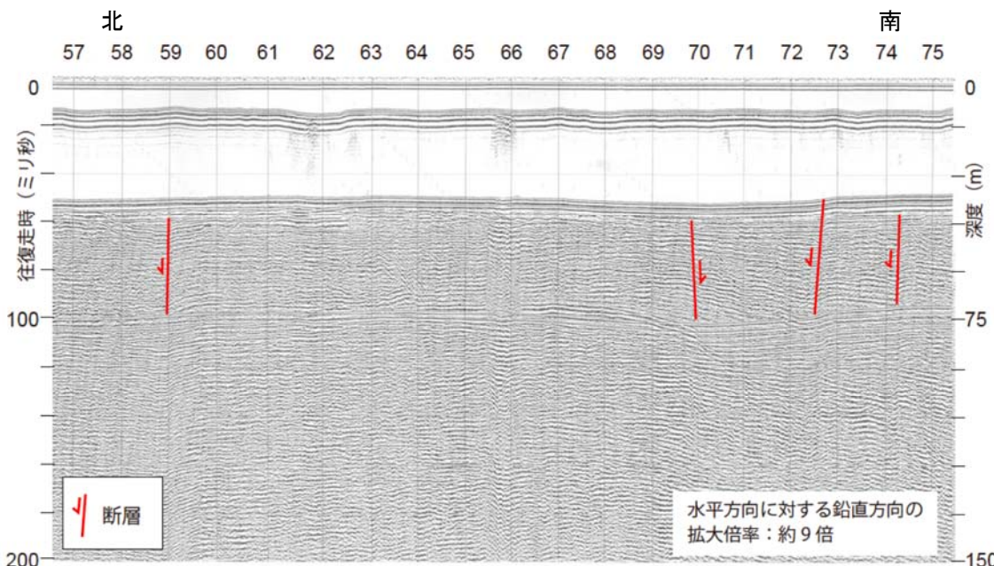
図5 宇土半島，宇城市三角町太田尾沖測線沿いのブーマーを音源とするショートマルチチャンネル音波探査(産業技術総合研究所ほか，2010 に加筆) (上)測線位置。(下)S6測線沿いの測位点57-75における重合断面(時間断面)。断面の位置は測線図(上図)に紫線で示す。
