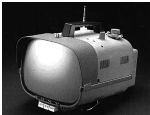
TV 8-301 8インチTV Tr 23石 Di 19石
