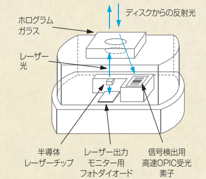
ホログラムレーザーの内部構造の一例
