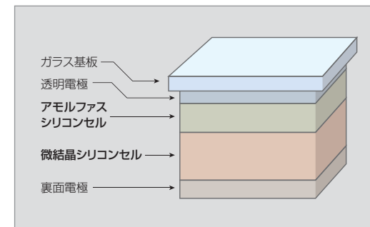
幅広い波長の光を2階層のセルでそれぞれ発電に利用する結晶薄膜タンデムセル太陽電池 (構造図)
