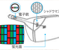
1972年 / 141C-401 水平電子銃で色ズレなし
