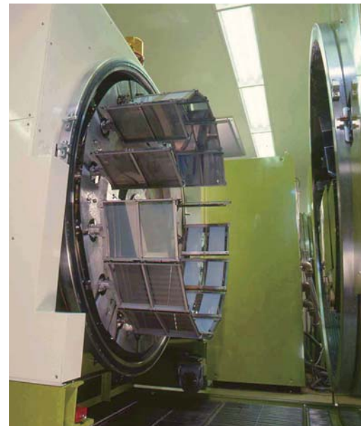
ガラスの基板に薄膜を高温で真空蒸着するELパネル蒸着装置
