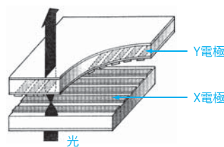
〈単純マトリクス駆動方式の構造〉
