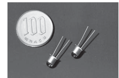
近赤外光と同時に緑色可視光を放射するガリウム砒素ダブル発光ダイオード(GLE-50G)
