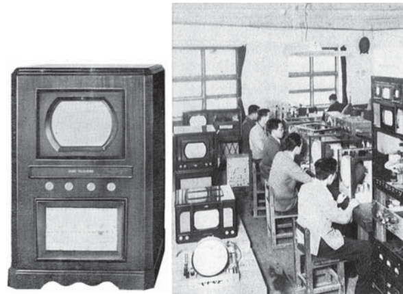
12型ブラウン管のグラント型テレビ試作機(1951年)(左) テレビの研究所(1952年)(右)
