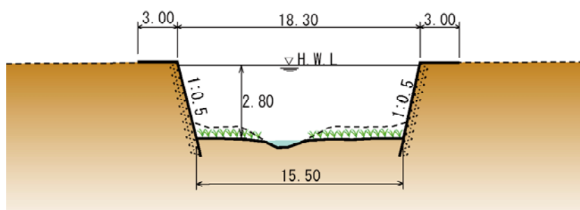
< 大和沢川上流工区代表横断面図 >
