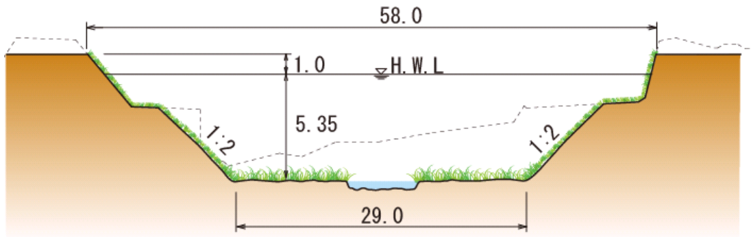
< 平川工区代表横断図 >
