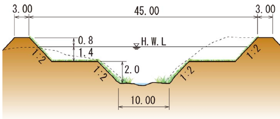
< 大和沢川上流工区代表横断面図 >
