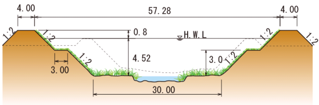
< 引座川工区代表横断図 >
