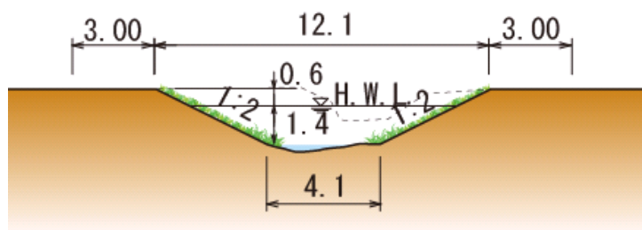
< 腰巻川工区代表横断面図 >
