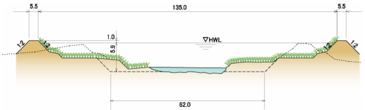
旧十川代表横断面図
