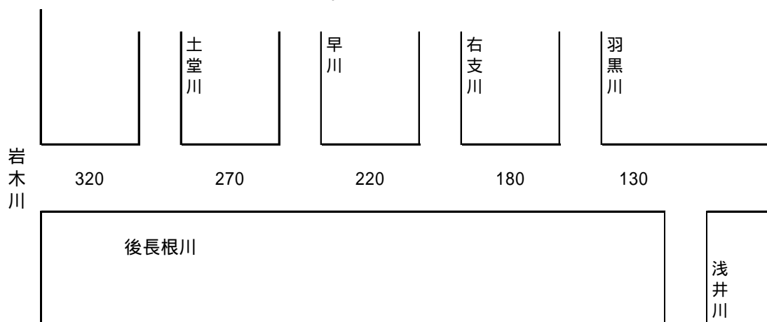
整備計画目標流量配分図( m 3 /s)
