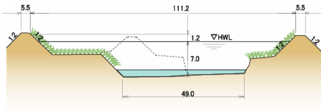
十川代表横断面図
