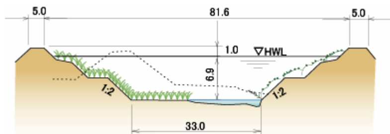
金木川代表横断面図
