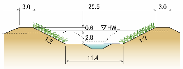
後長根川代表横断面図
