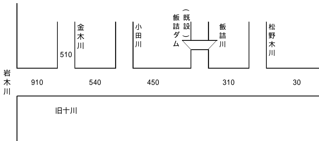
整備計画目標流量配分図( m 3 /s)
