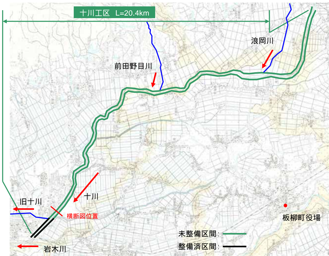
整備事業位置図(十川)
