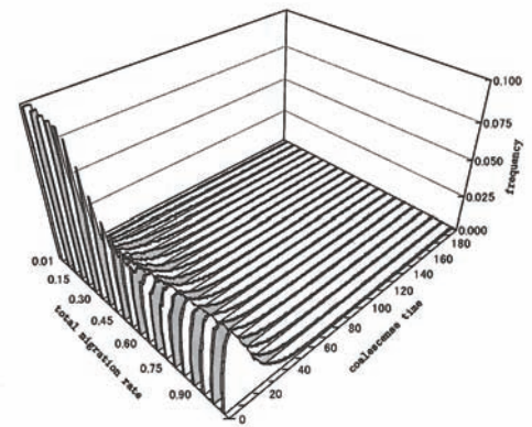
Coalescence time の分布
