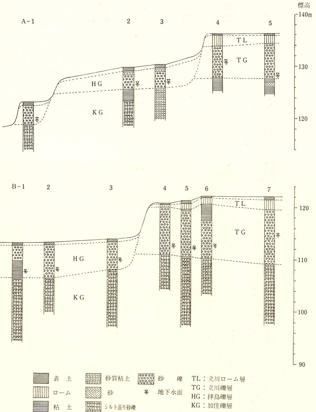
第7図 ボーリング柱状図(1)
