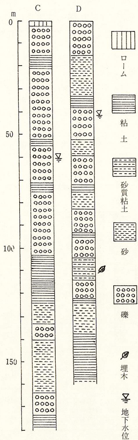
第8図 ボーリング柱状図(2)
