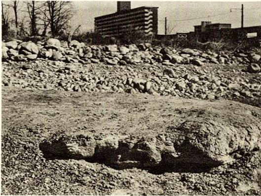
2. 多摩川五日市線鉄橋下の露頭 下から加住礫層の砂・シルト部分、 同礫層、最上部は多摩川河床礫
