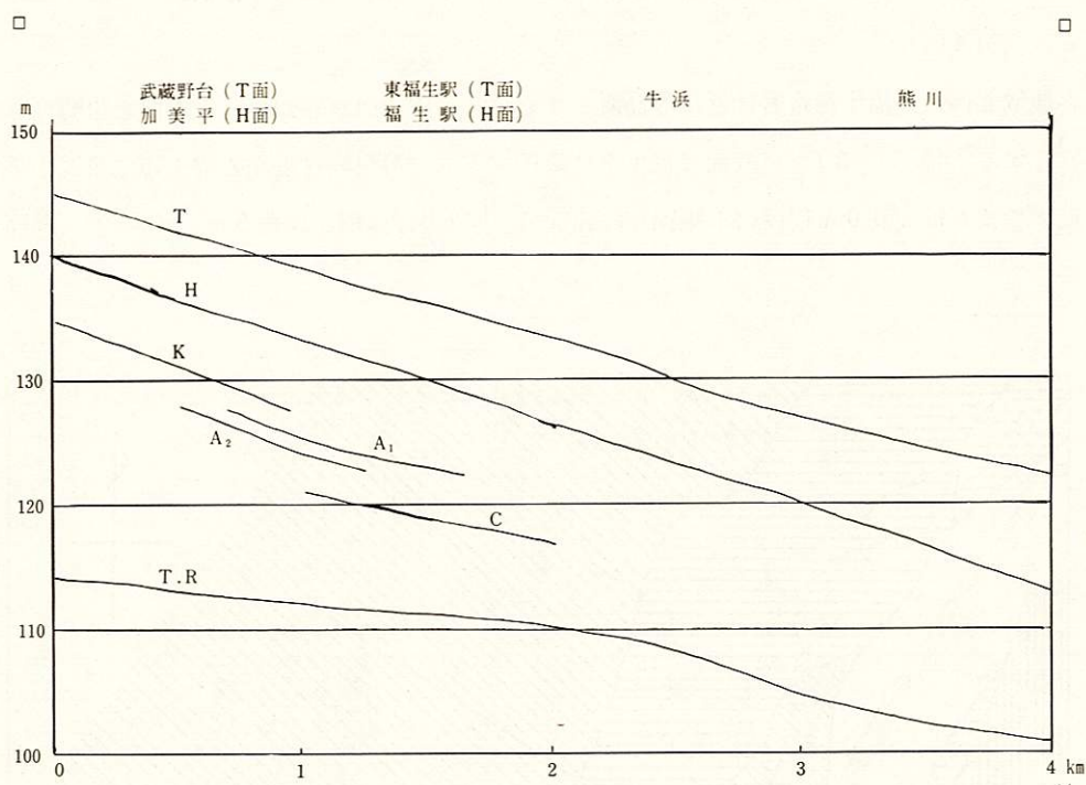
第4図 段丘面の勾配
