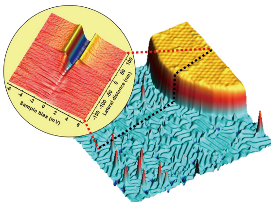
超伝導金属界面での近接効果。Si 基板上的 1 原子層 Pb (水色、常伝導相) と Pb 薄膜 (黄色、超伝導相) の界面近傍で測定されたトンネル分光スペクトルから、超伝導特性が界面から 40nm の領域にわたって染み出していることが観察されている。
