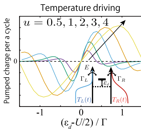
左右のリード温度 T_L(t) , T_R(t) を時間変化させることで生じる断熱ポンピング一周あたりの輸送電荷。挿入図は系の模式図。 U はクーロン相互作用の大きさ、 \Gamma_L = \Gamma_R = \Gamma/2 はリードとの結合の強さ、 \epsilon_d は量子ドットのエネルギー準位、 u = U/\Gamma は無次元化したクーロン相互作用パラメータ。
