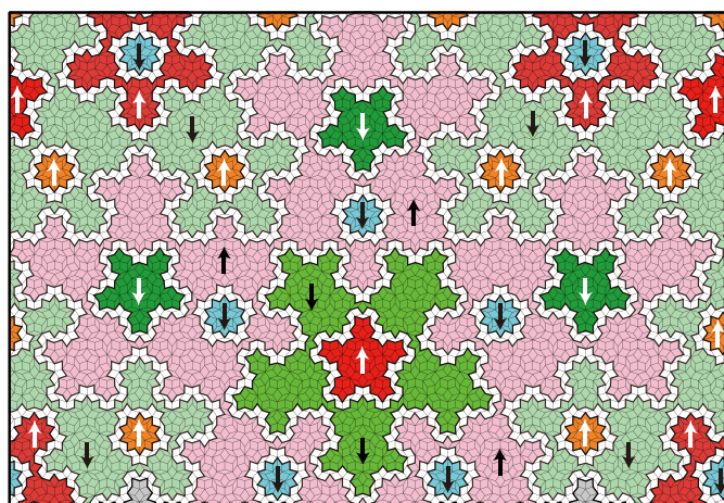
二次元ペンローズ格子上の half filled ハバード模型の基底状態の反強磁性秩序の磁区。フラクタル構造を示している。
