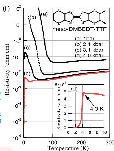
図1. 新規有機超伝導体: (i) モット型 \kappa -ET 2 Cu(NCS) 2 の単結晶と (ii) 電荷秩序型 \beta -( meso -DMBEDT-TTF) 2 PF 6 の電気抵抗の圧力依存性。
