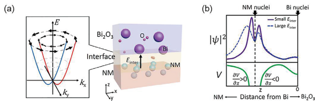
非磁性金属 (NM)/ 酸化ビスマス ( \text{Bi}_2\text{O}_3 ) 界面状態のラシュバ分裂の見積り。NM/ \text{Bi}_2\text{O}_3 界面のラシュバパラメータの大きさと符号は、NMの種類 (Cu, Ag, Au) に依存する。これは、界面状態の電荷密度 |\psi^2| の非対称性が、NMと \text{Bi}_2\text{O}_3 の仕事関数の差で決まる内部電場 E_{\text{inter}} に依り変調される結果であることが明らかになった。(a)NM/ \text{Bi}_2\text{O}_3 界面とラシュバ分裂の概略図。(b) NM/ \text{Bi}_2\text{O}_3 界面近傍の |\psi^2| と電位 V の空間分布。
