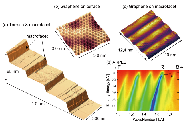
(a-c) 傾斜 SiC 基板を Ar 雰囲気中で熱分解することによって形成されたステップ・テラス構造の STM 像 (a) と、それらの上の 2 次元および 1 次元的なナノ周期構造をもつグラフェンの STM 拡大像 (b,c)。基板表面 (a) には、SiC(0001) テラス面とそこから 28 度傾いたマクロファセットが共存し、テラスの一部 (b) とマクロファセット上 (c) に単層グラフェンができる。(d) 1 次元ナノ周期構造グラフェンからのディラックバンドの角度分解光電子分光スペクトル。複数のレプリカバンドが観測され、ディラックバンドのドーピング量はテラスに比べて低い。
