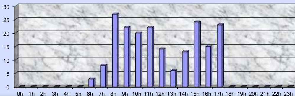
Movimento Horário no Dia da Hora-Pico de Passageiros Simultâneos 20/09/2014
