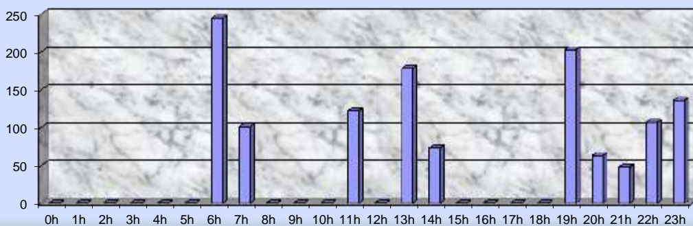
Movimento Horário no Dia da Hora-Pico de Passageiros Simultâneos 10/02/2014
