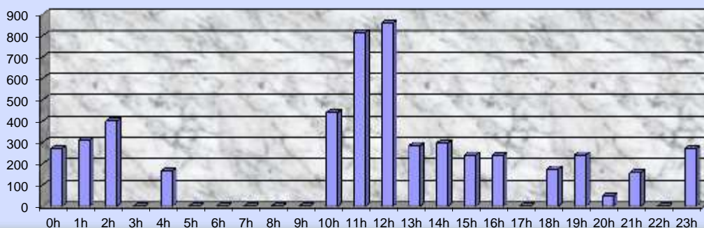
Movimento Horário no Dia da Hora-Pico de Passageiros Simultâneos 31/10/2014
