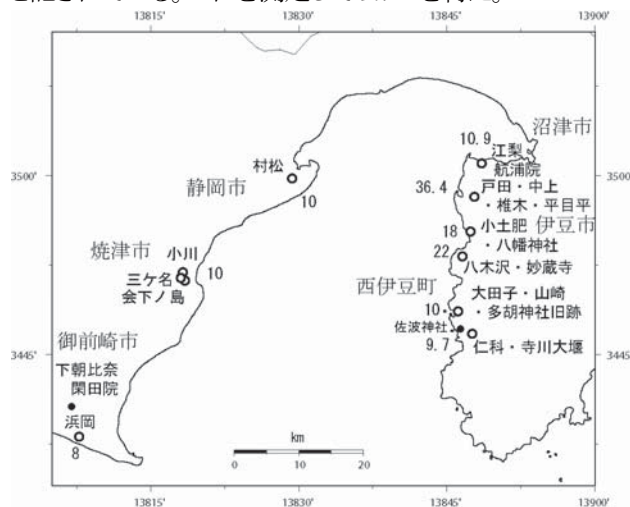
図 明応東海地震(1498)の津波遡上高さ(m)
