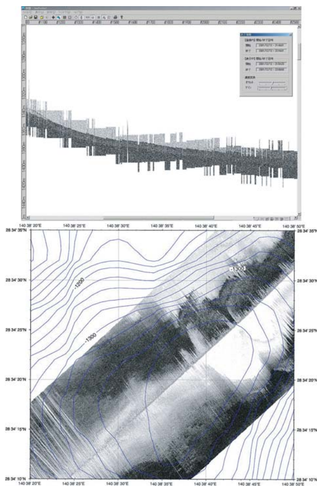
図5 深海曳航式「わだつみ」による水曜海山カルデラ底のサブボトムプロファイラー(上図)とサイドスキャンソナーイメージ(下図)の結果。海山の地形変化に対応して曳航深度を細かく変化させたためにイメージの解像度があまり高くない。 Fig. 5 Sub-bottom profiles (top) and side scan sonar intensity images (bottom) obtained by a deep towed WADATSUMI survey. Quick changes in towing depth to follow the topography resulted in poor images.
