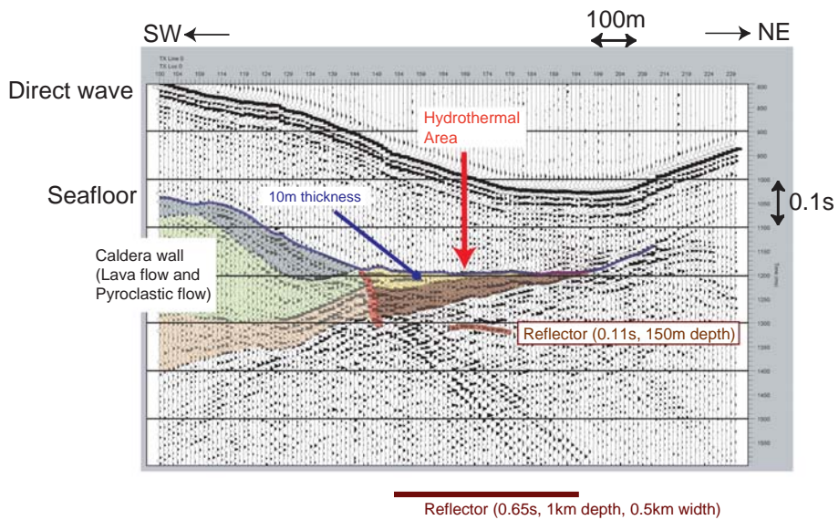
図4 水曜海山のカルデラを南西-北東方向に横切る地震波反射断面図。堆積層が南西側ほど厚くなる非対称な構造になっている。 Fig. 4 Seismic reflection image across the Suiyo seamount in SW-NE direction. Difference in thicknesses of two layers beneath the caldera center exists between the SW and NE sides.
