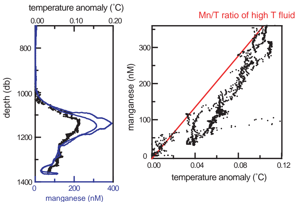
図9 現場化学分析計GAMOS-II (Okamura et al., 2001) により得られた熱水ブルーム中のマンガン濃度とCTDセンサにより得られた温度異常。鉛直プロファイル(左図)と両者の関係(右図)を示した。マンガン濃度/温度異常の比はブルーム中心層では高温熱水における比(赤線で示した)とほぼ一致するが、その他の層ではこれよりも明らかに低くなっている。
