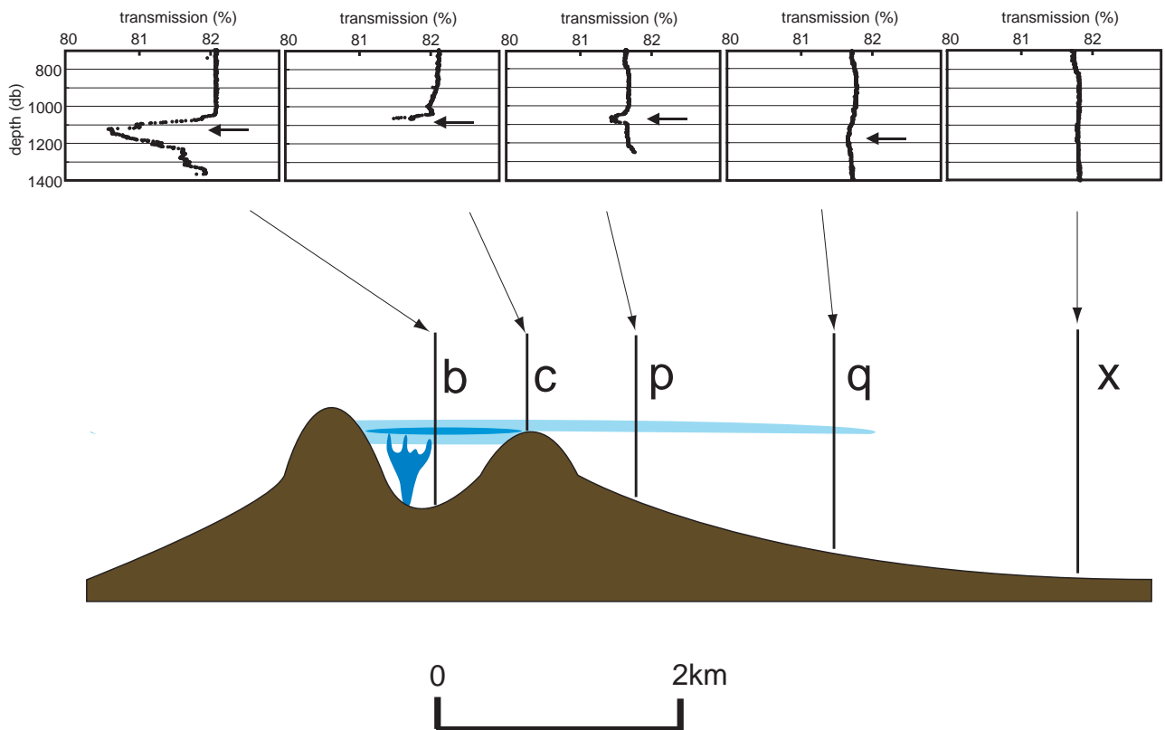
図8 水曜海山カルデラ内外の水塊の透過度異常の鉛直プロファイル。熱水ブルームはカルデラ内で強くカルデラから離れるにつれて急激に弱くなる分布を示した。
