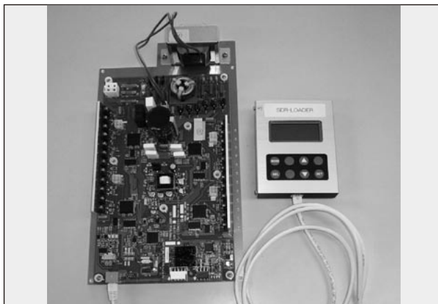
図 20 4 台運転 DC-FFU コントロール基板
