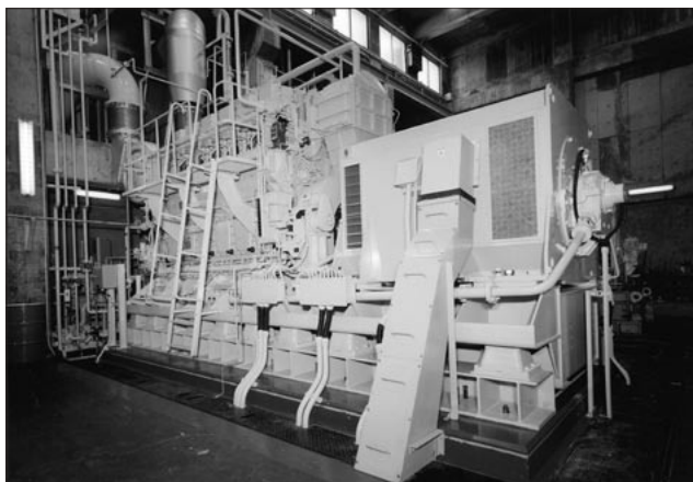
図 19 2,500 kVA ディーゼル発電装置
