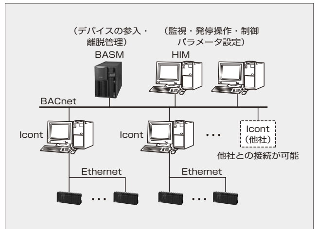
図 18 BACnet 監視システム構成
