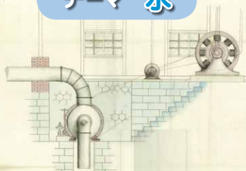
水力発電所の発電機と 水車の図面
