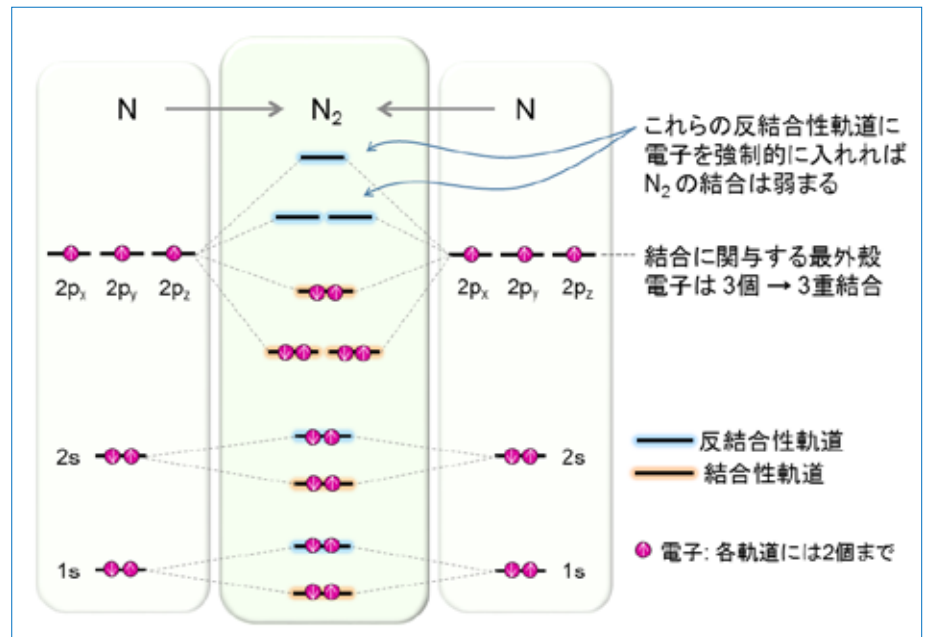
⑤ 窒素分子の電子配置と安定性。窒素原子 (N) の場合、原子核の周りに7個の電子 (●) が存在し、それらが決められた軌道上 (1s, 2s, 2p x , 2p y , 2p z ) を回っている。N 原子同士が近づくと、軌道は、よりエネルギーの低い安定な軌道 (結合性軌道) と不安定な軌道 (反結合性軌道) に分かれる。エネルギー準位の低い軌道から順に電子が2個まで入るので、N 2 の場合は、中央の縦列に示すように、最上位の反結合性軌道のみが空の3重結合状態で安定化する。これに外部から強制的に電子を付加すると、それらの電子は反結合性軌道にしか入ることが出来ず、N 2 結合は弱くなり解離しやすくなる。
