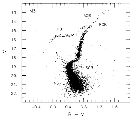
図1 球状星団M3の Hertzsprung-Russell(HR) 図 9) 。AGB：漸近巨星分枝，RGB：赤色巨星分枝，SGB：準巨星分枝，MS：主系列，HB：水平分枝。
