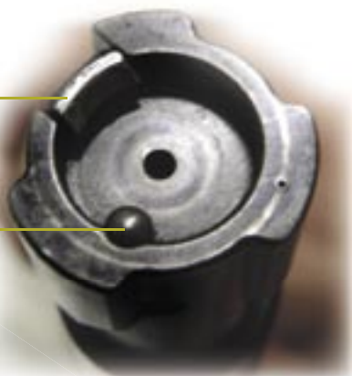
Hlava závěru s uzamykacími ozuby
