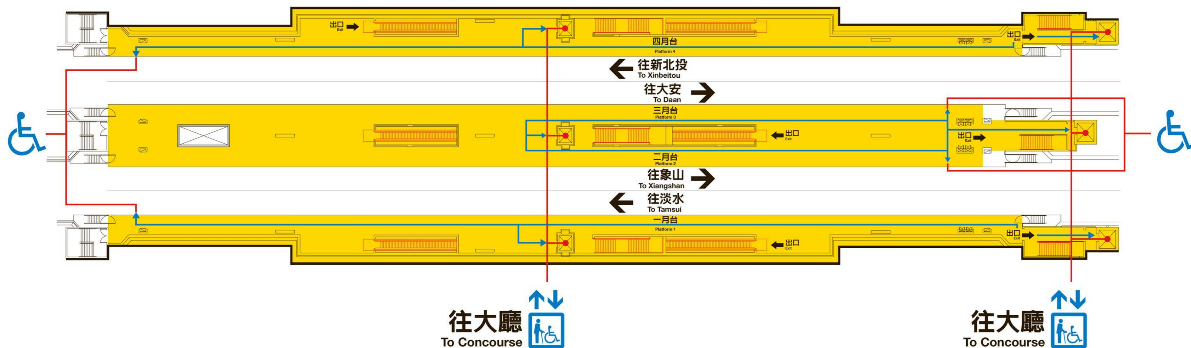
月台層平面圖 Platform Level
