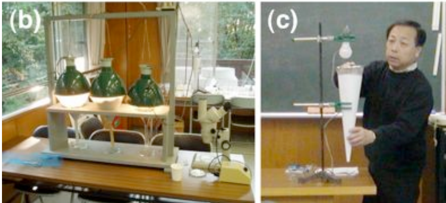
図7.2 ツルグレン装置：(a) ツルグレン装置の自作例，(b) ツルグレン装置（左）と実体顕微鏡（右），(c) 自作したツルグレン装置（写真提供：愛知県農業総合試験場 瀧勝俊）
