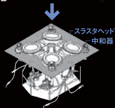
「はやぶさ」は4基のイオンエンジンを搭載している。イオンエンジンAは打ち上げ直後に動作不安定で運用を休止していた。イオンエンジンBは電圧上昇のため運用休止中（2007年4月以降）。2009年11月3日、中和器の電圧が上がり、動作中のイオンエンジンDが異常停止した。イオンエンジンCは停止中だが、稼働することを確認している
