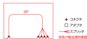
[32]分岐小型スプリッタモジュール (型番 32SPM[B])
