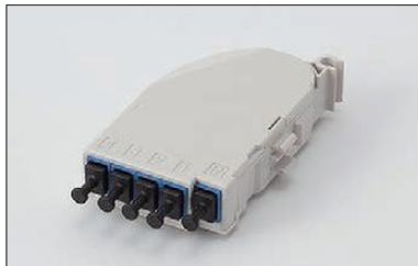
[4]分岐小型スプリッタモジュール (型番 4SPM[B])
