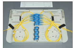
コネクタトレイFOタイプ (FOコード用)
