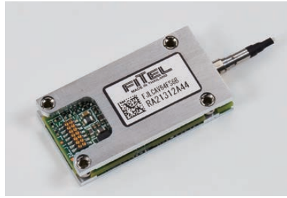
波長可変光源 MicroITLAモジュール
