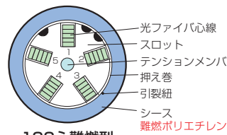
100心難燃型
