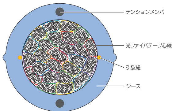
ケーブル断面図
