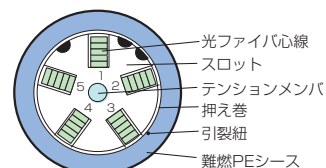
断面構造
