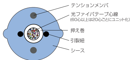
ケーブル断面図
