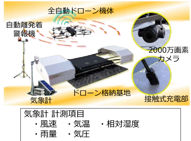
図-4 全自動ドローンシステム構成図
