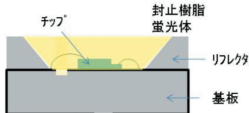
図3 LEDの構造
