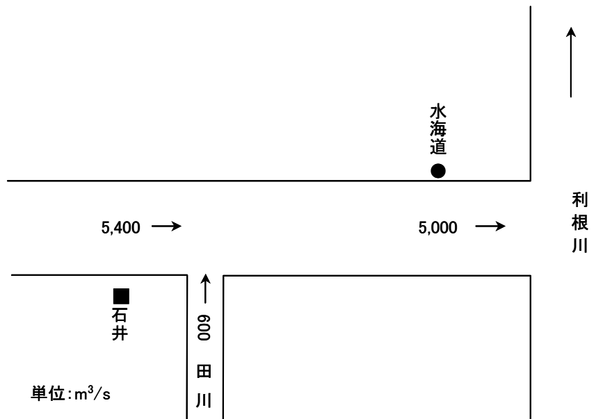
鬼怒川計画高水流量図
