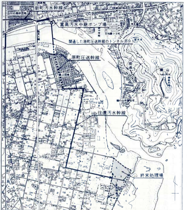
公共下水道事業計画図(一部)
