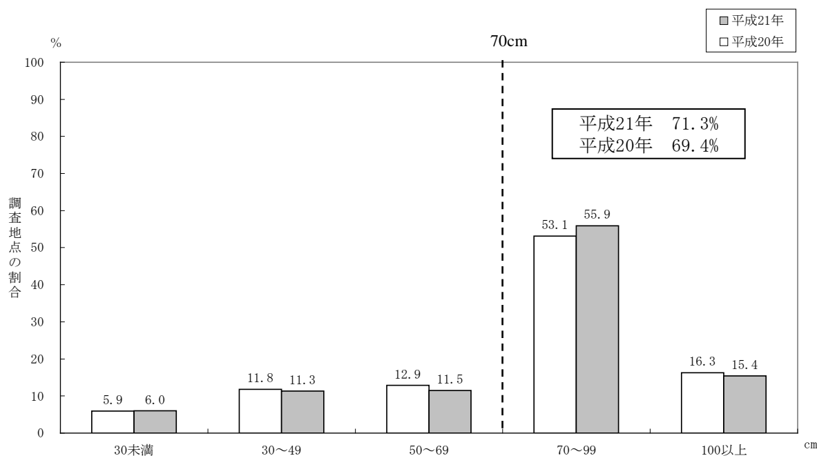
図-26 透視度（年平均値）のランク別割合
