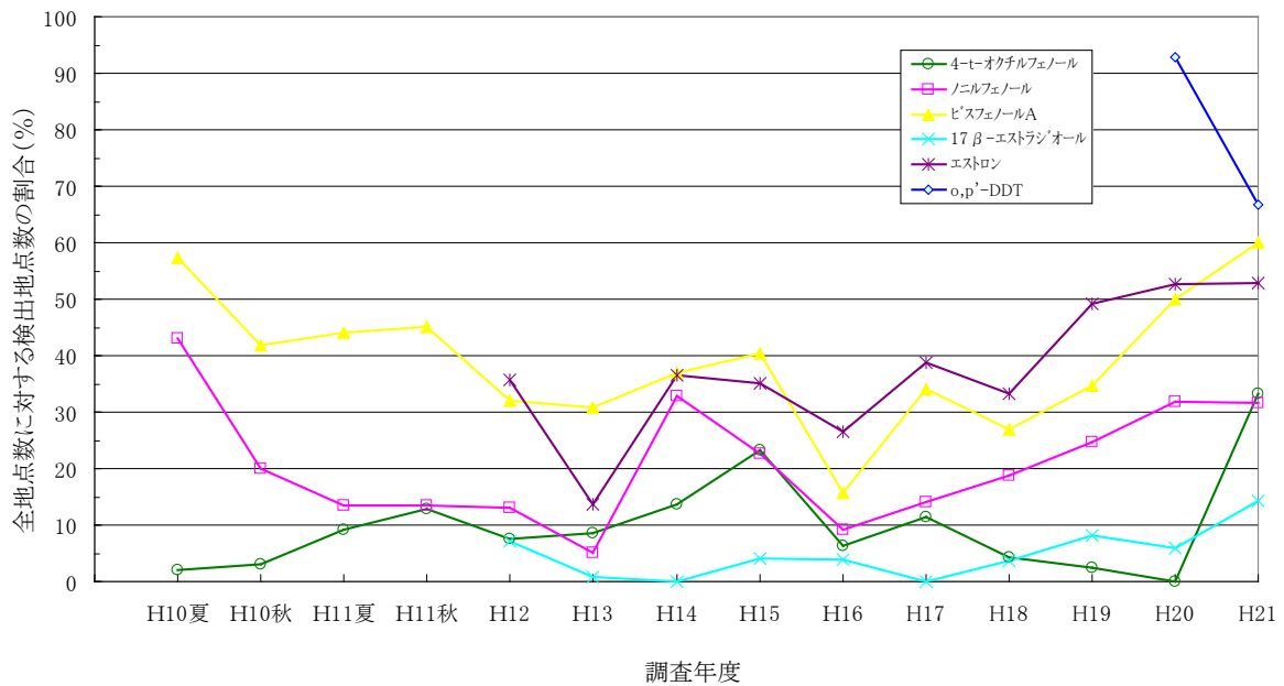
図-51 内分泌かく乱化学物質に対する検出地点数の割合 (%) の推移
