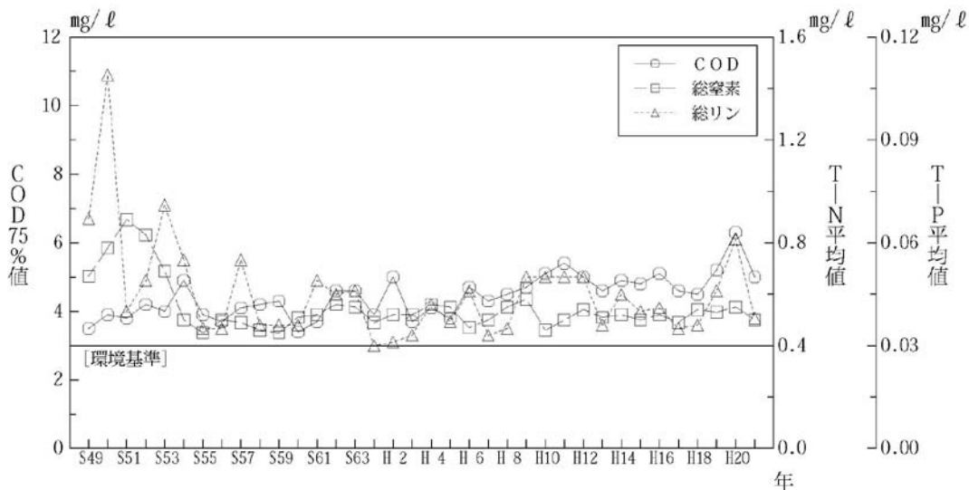
図-22(5) 主要湖沼代表地点における水質の経年変化 宍道湖No.3:湖心 (湖沼A, III)
