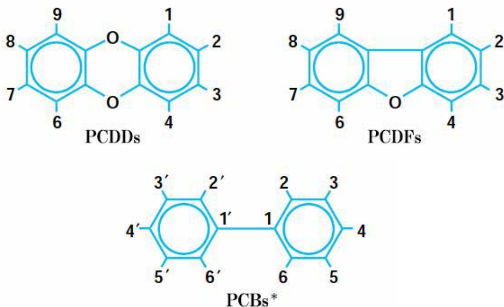
図-46 ダイオキシン類の構造図
