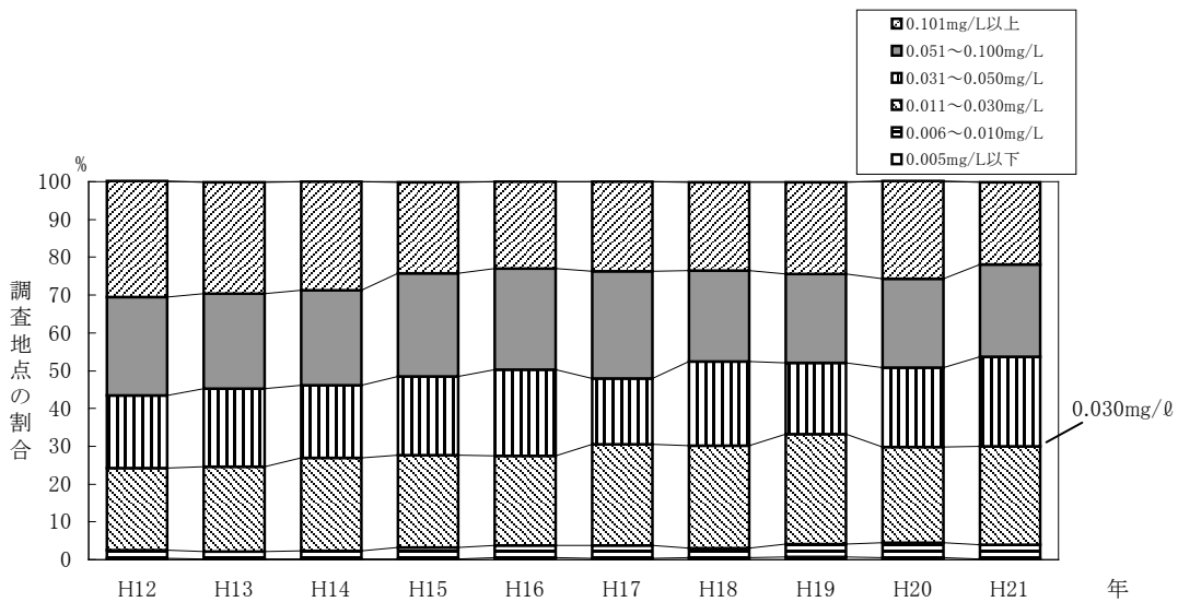
図-18(3) 総リン平均値ランク別割合の経年変化 (河川)
