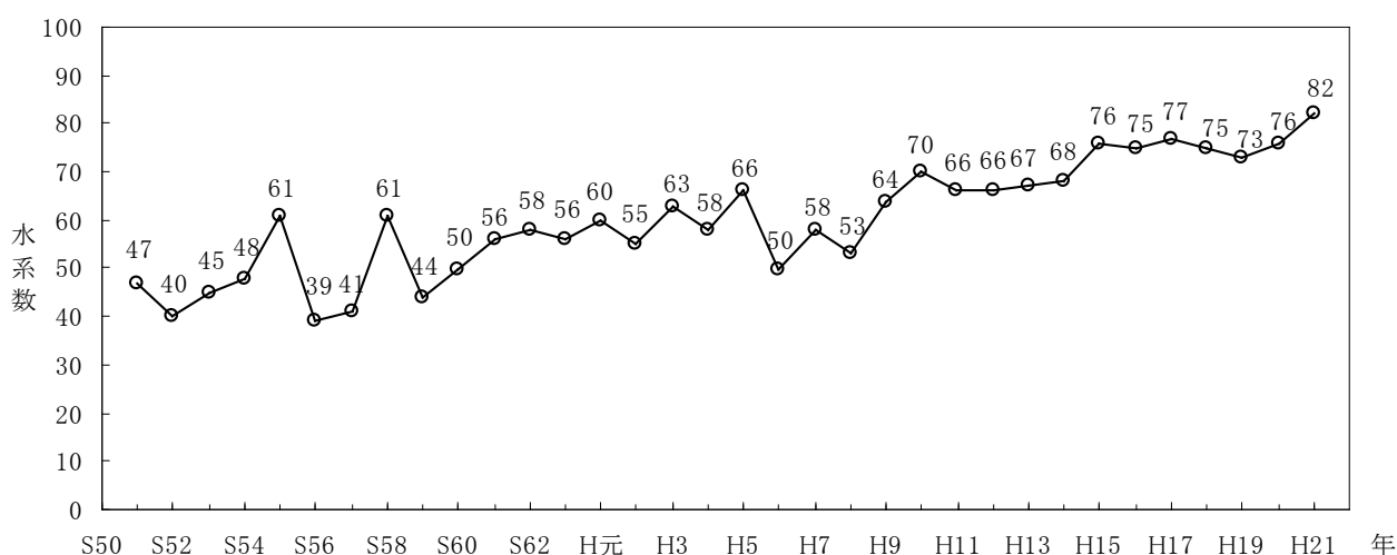
図-14 すべての調査地点が環境基準を満足している水系数の経年変化(全国)
