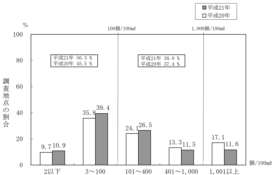
図-24 糞便性大腸菌群数（年平均値）のランク別割合
