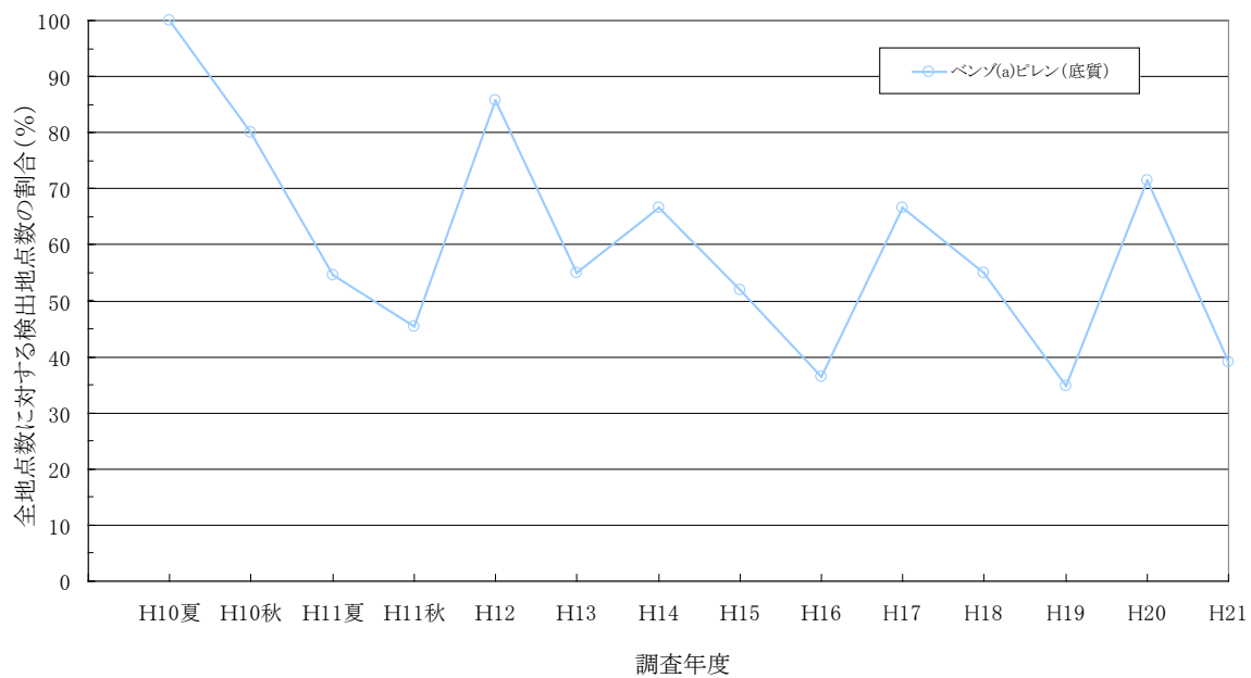
図-50 ベンゾ(a)ピレンに関する全調査地点数に対する 検出地点数の割合 (%) の推移
