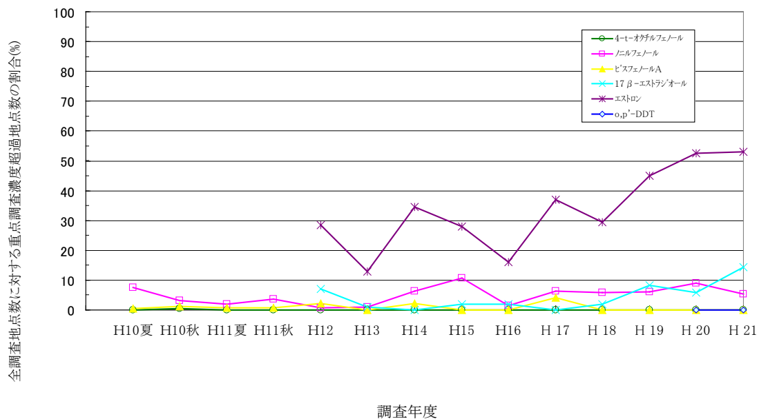
図-52 内分泌かく乱化学物質に関する全調査地点数に対する重点調査濃度超過地点数の割合 (%) の推移
