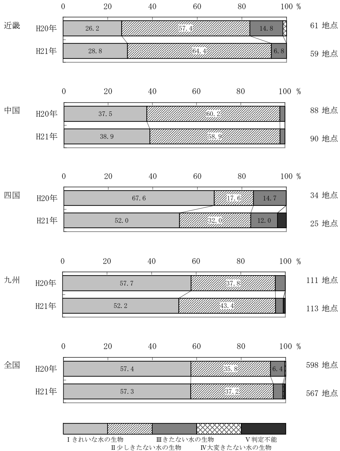
図-43(2) 水生生物による水質調査結果（地点割合）
