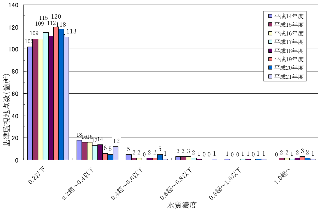
図-48 平成14年度～平成21年度水質ダイオキシン類調査（基準監視地点）濃度ヒストグラム
