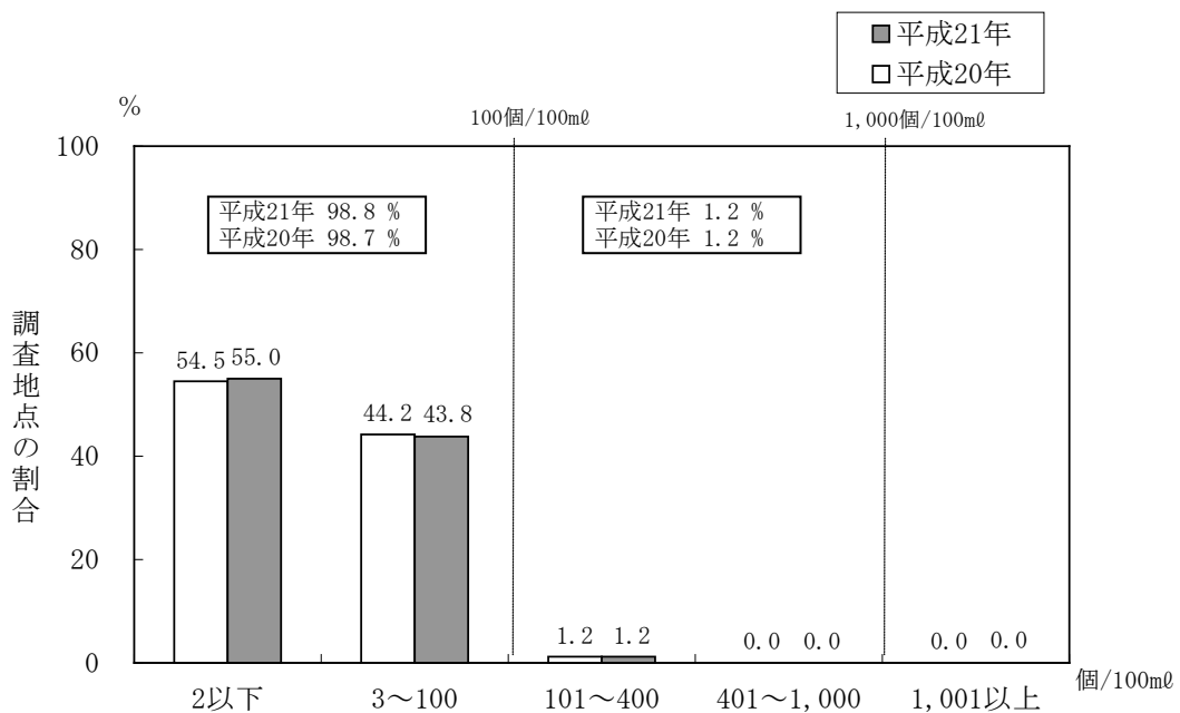
図-25(2) 糞便性大腸菌群数のランク別割合 (湖沼等の表層)
