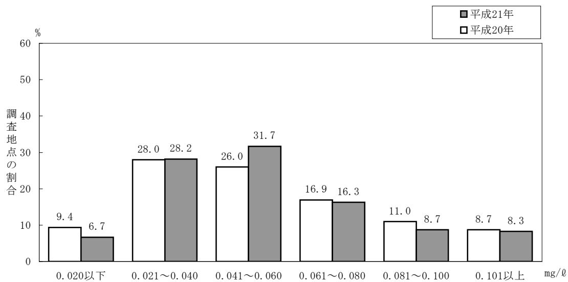
図-23 トリハロメタン生成能（最大値）のランク別割合
