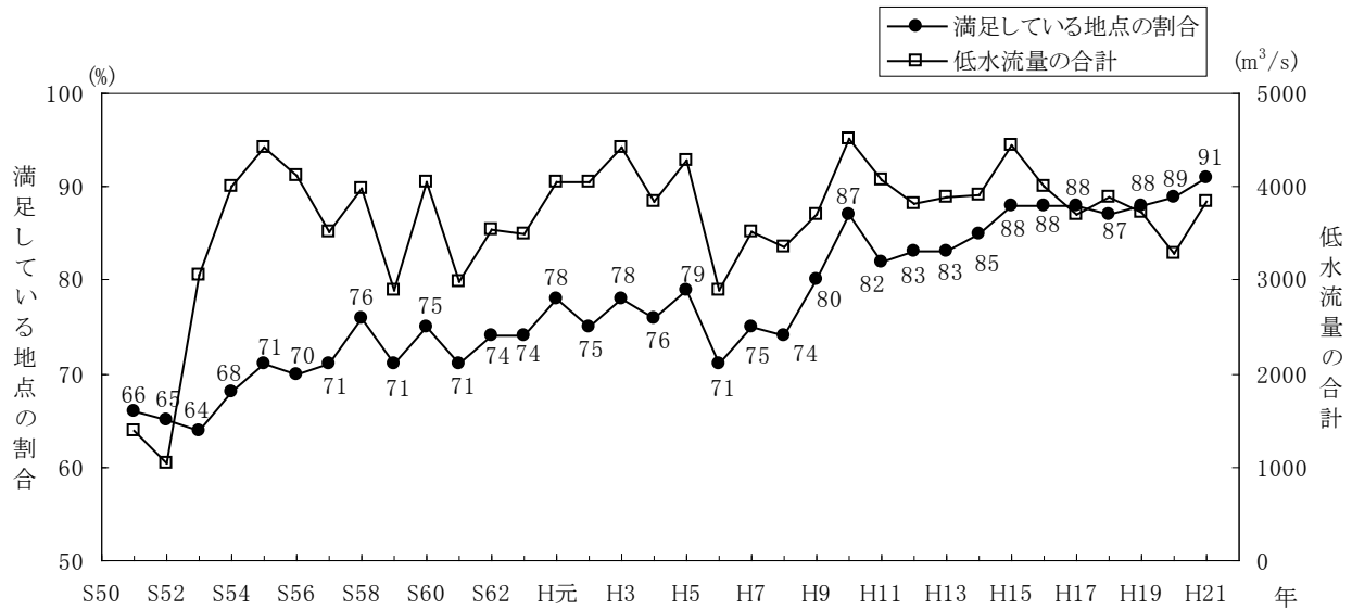
図-9(2) 一級河川(湖沼及び海域も含む。)において環境基準を満足している地点の割合と低水流量の合計の経年変化(全国)
