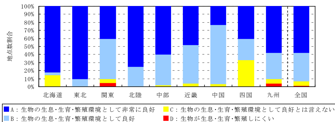
図-37 年間の地点評価のランク別割合 (豊かな生態系の確保)
