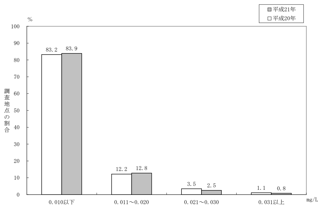
図-28 全亜鉛（年平均値）ランク別割合
