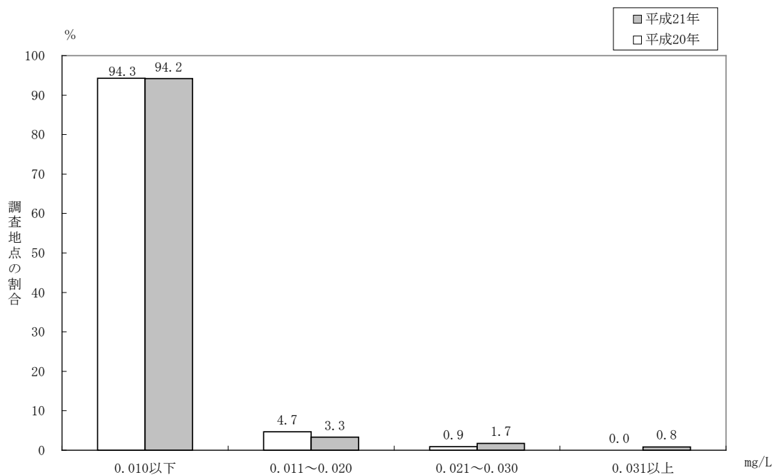
図-29(2) 全亜鉛 (年平均値) ランク別割合 (湖沼等)
