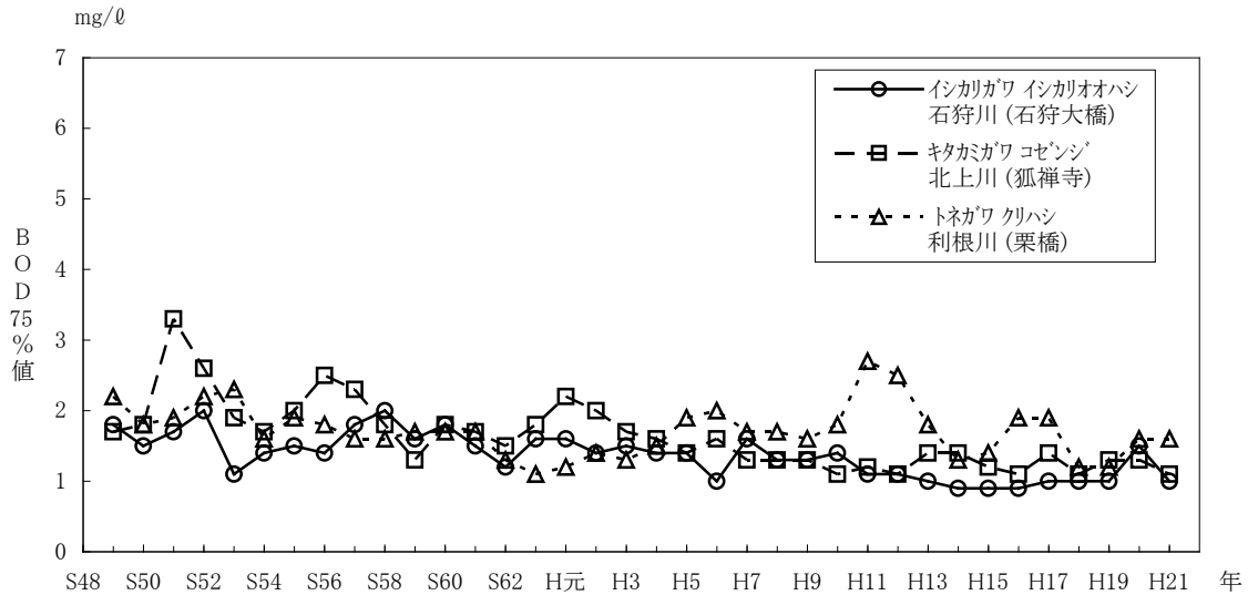
図-20(1) 主要河川の代表地点におけるBOD75%値の経年変化
