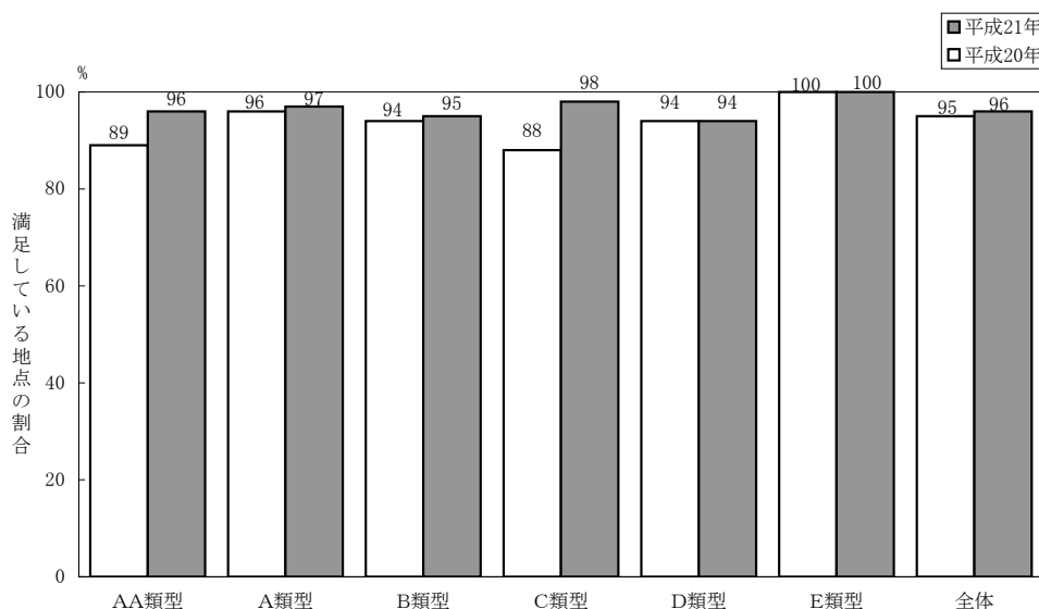
図-11(1) 一級河川における環境基準を満足している地点の類型別割合 (河川)
