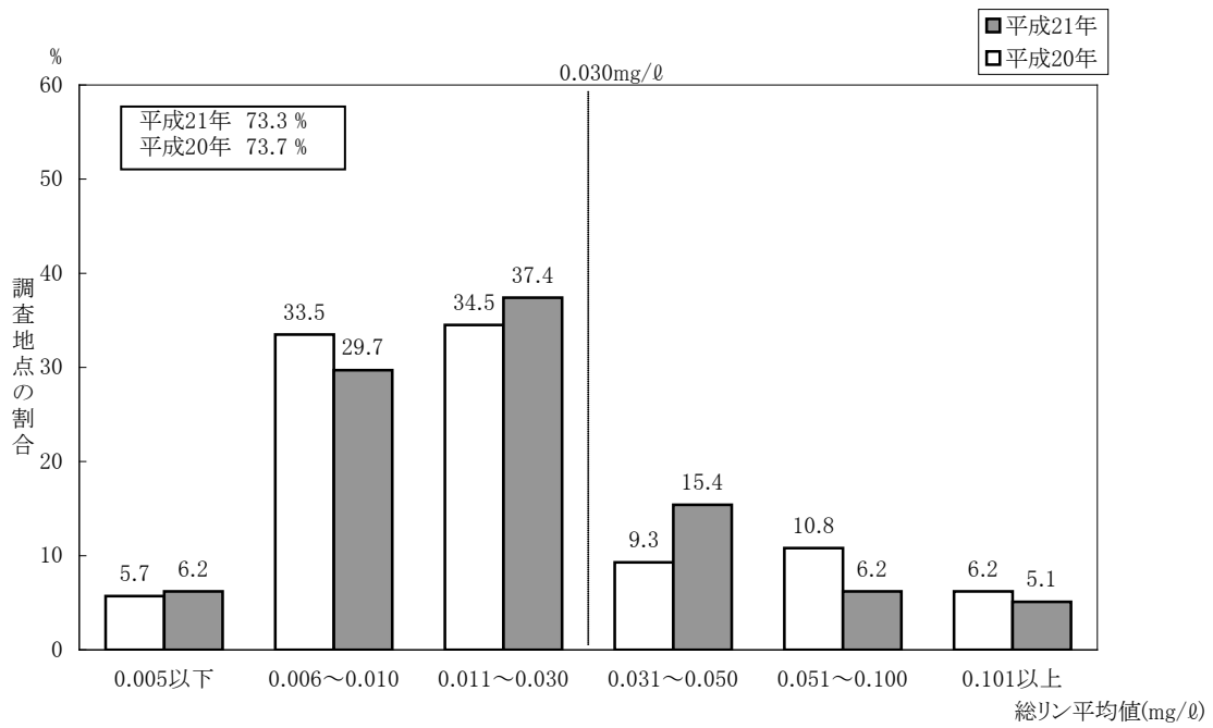
図-17(3) 総リン平均値ランク別割合 (湖沼等)
