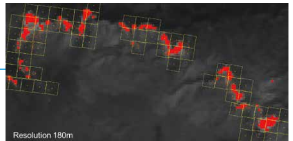
ASTERデータをもとにしたCIRCの火災検知シミュレーション画像 Image of CIRC fire detection simulation based on ASTER data
