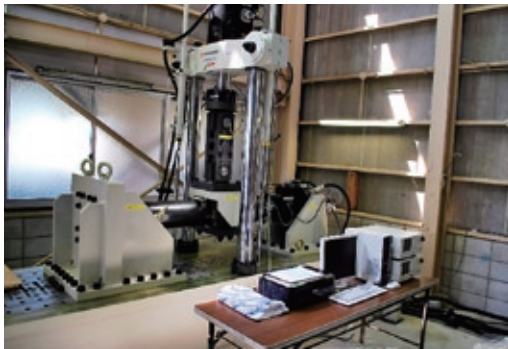
◀ 300kN 油圧サーボ2軸疲労試験装置 The 300kN hydraulic servo test system
