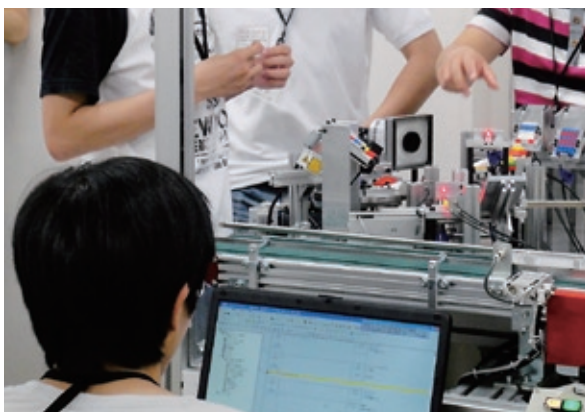
▲ 情報科学実験の様子：製造ラインの制御プログラムの開発 Computer Engineering Experiments on Development of Control Software for Production Line
