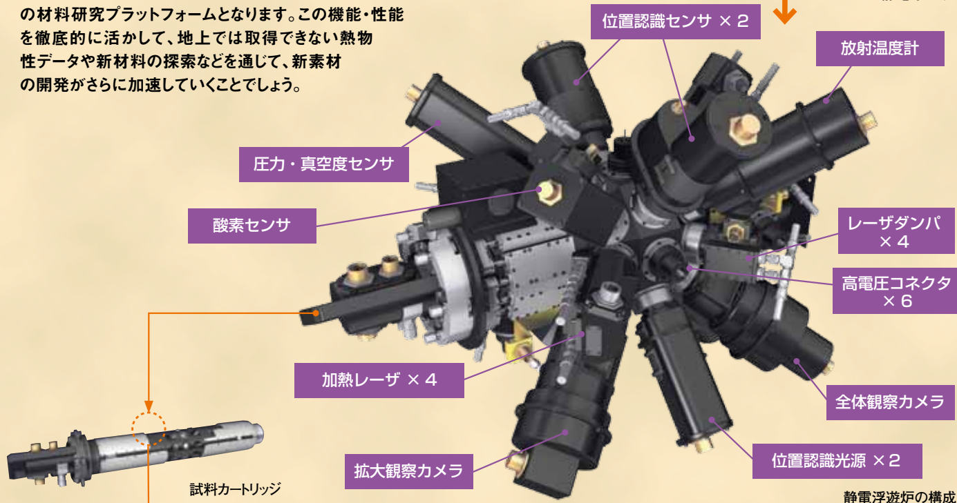
静電浮遊炉
