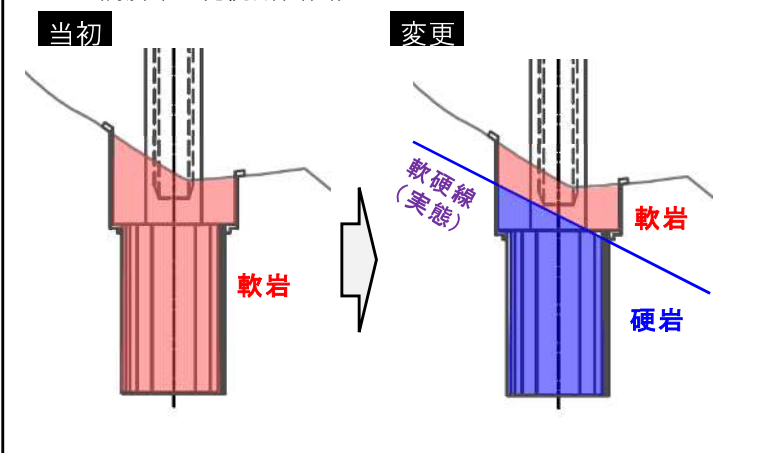
<P4橋脚(基礎杭断面図)>
