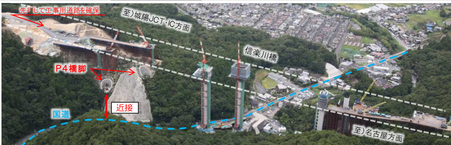
①傾斜地における橋梁工事
