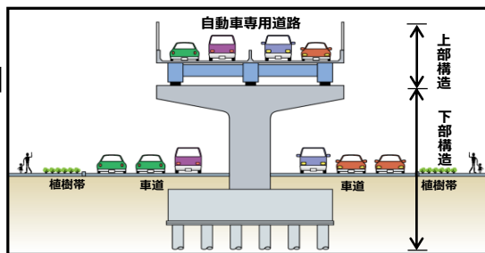
標準断面図
