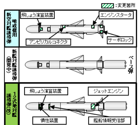
12式地对艦誘導弾（改）及び哨戒機用新空対艦誘導弾のファミリー化イメージ
